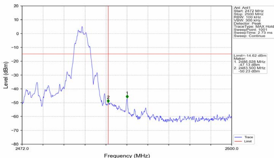
2M_HCH_2480MHz_Ant1_NTNV
