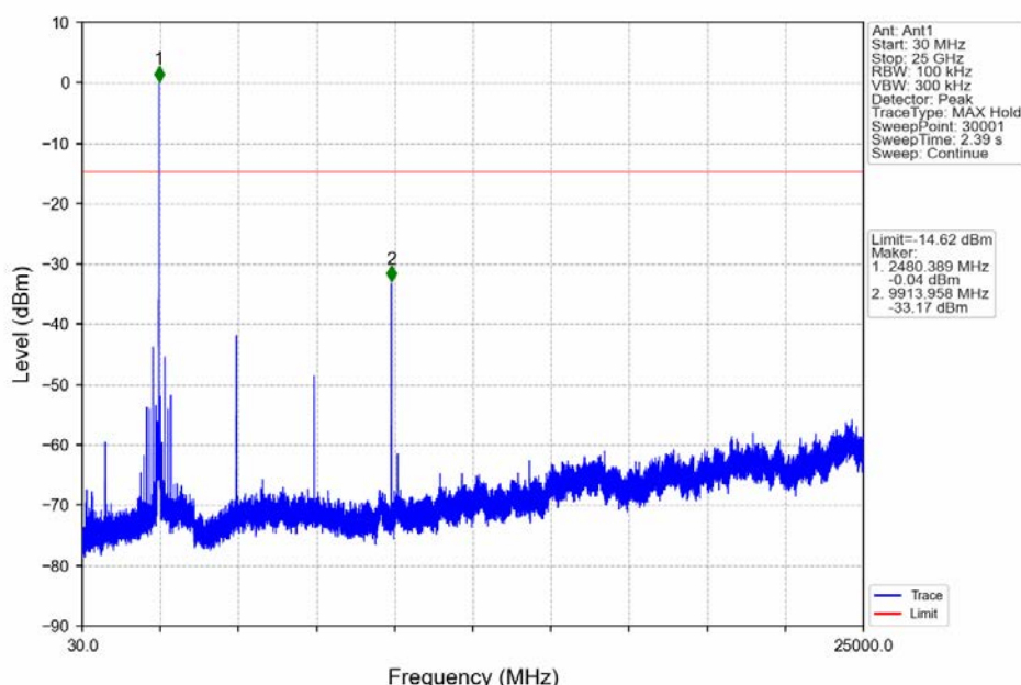
2M_HCH_2480MHz_Ant1_NTNV
