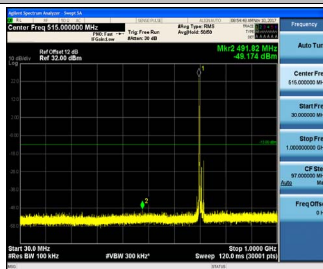
Band17 10MHz QPSK 23780 1RB#0
