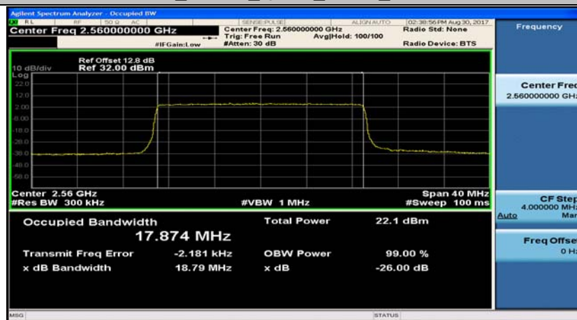
Band7_20MHz_16QAM_21350_100RB#0
