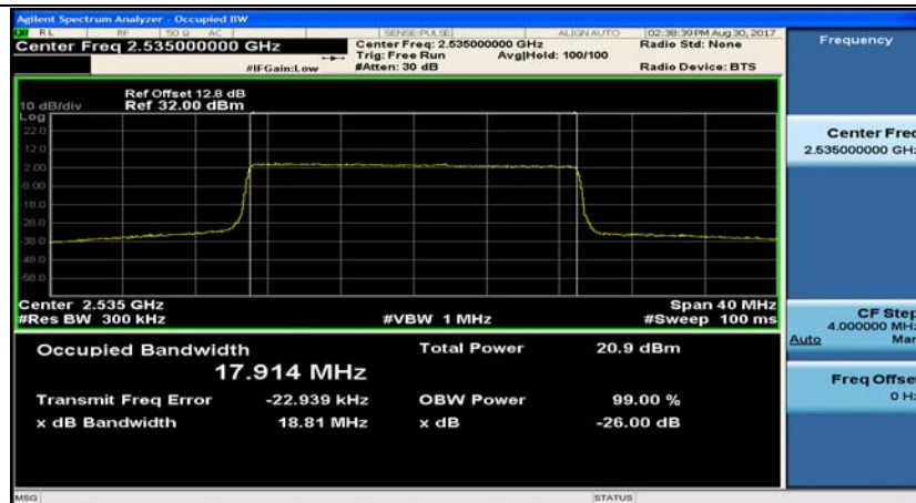
Band7_20MHz_QPSK_21350_100RB#0
