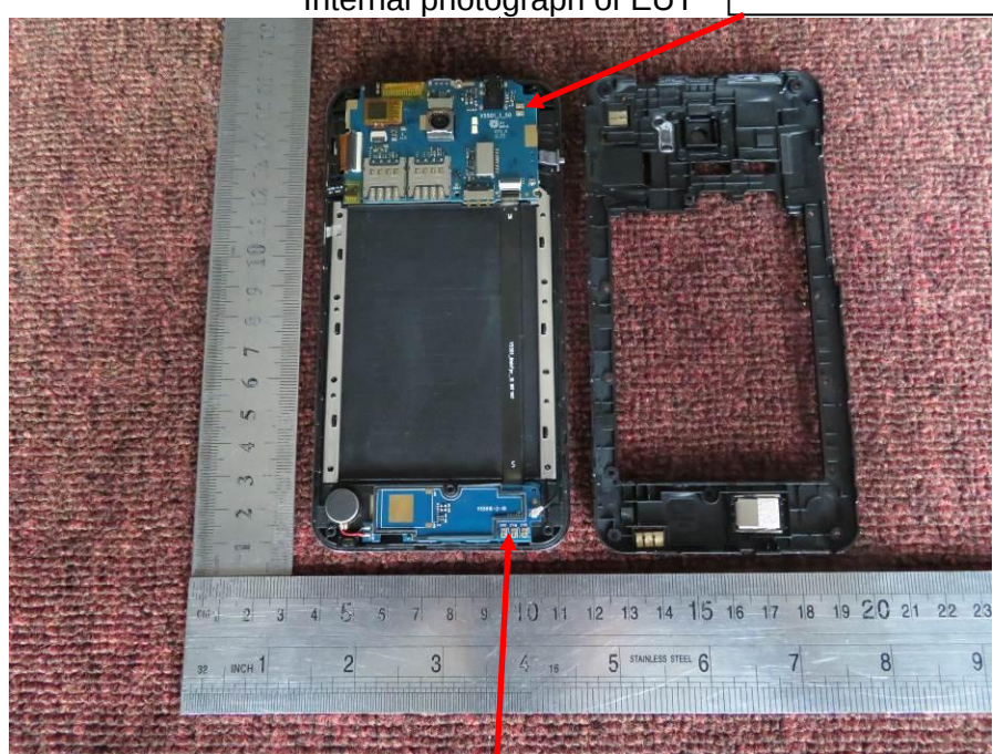
GSM/WCDMA Antenna
