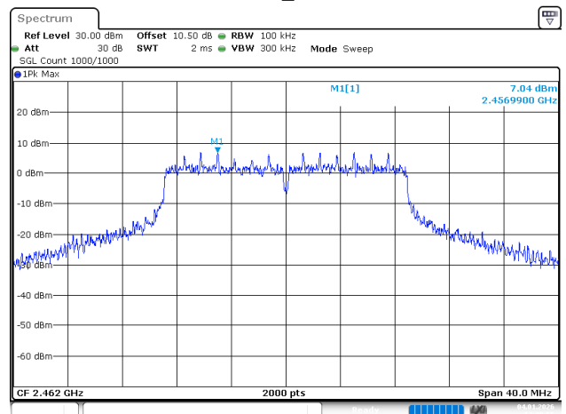
802.11n20_2462MHz
