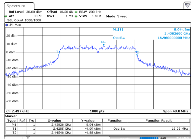
802.11g_2437MHz
