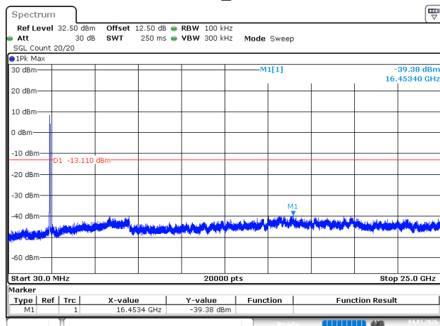
802.11n20_2412MHz
