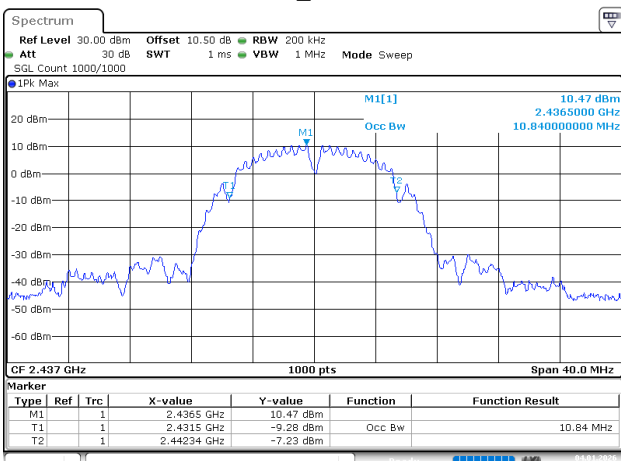
802.11b_2437MHz
