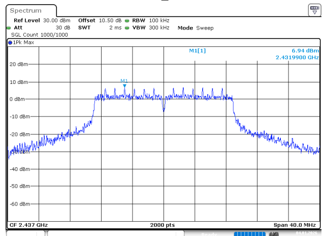
802.11n20_2437MHz
