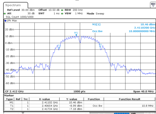
802.11b_2412MHz
