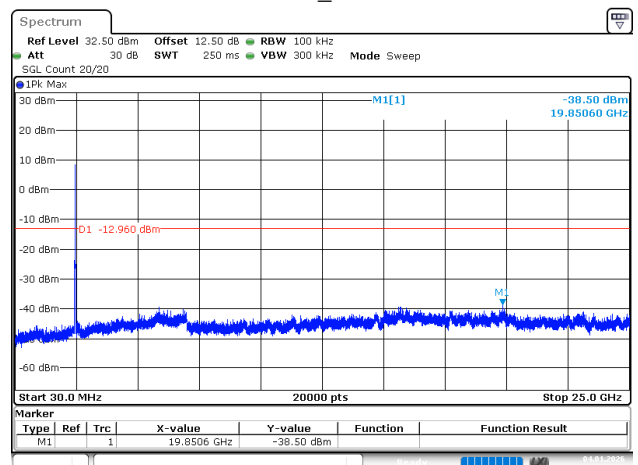
802.11n20_2462MHz
