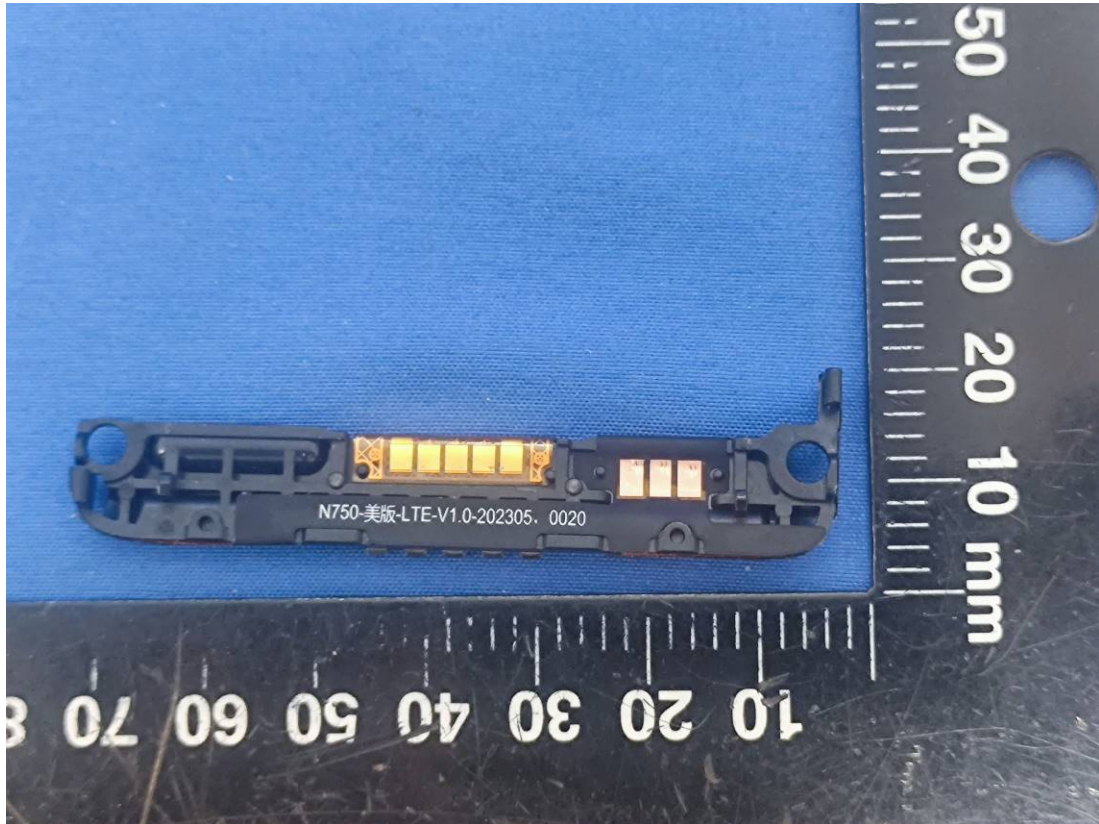
LTE Antenna
