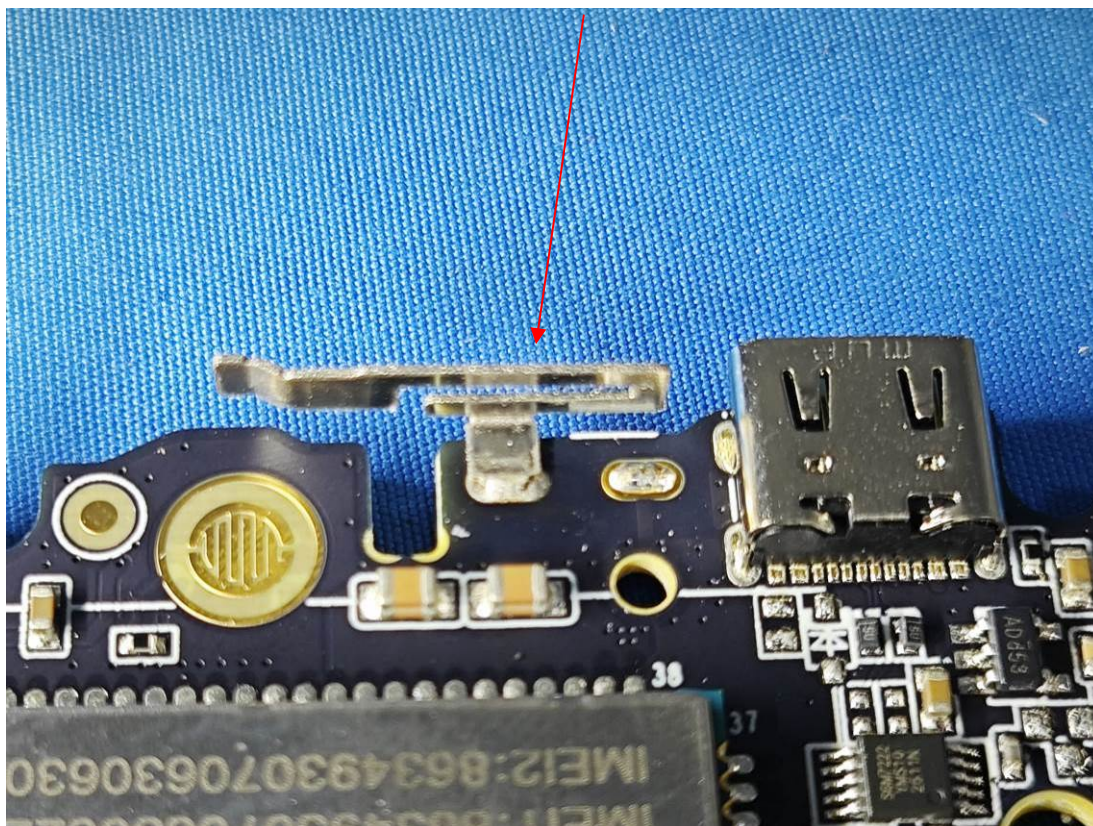
Bluetooth&Wifi Antenna
