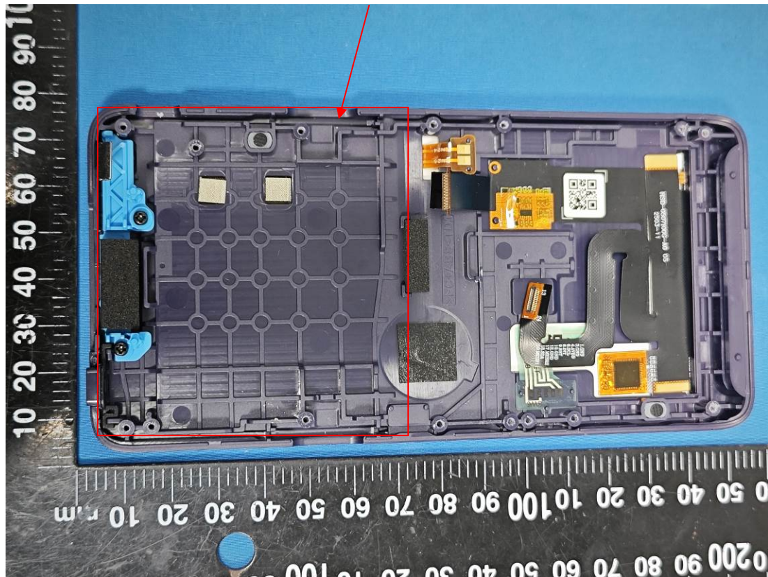
NFC Antenna
