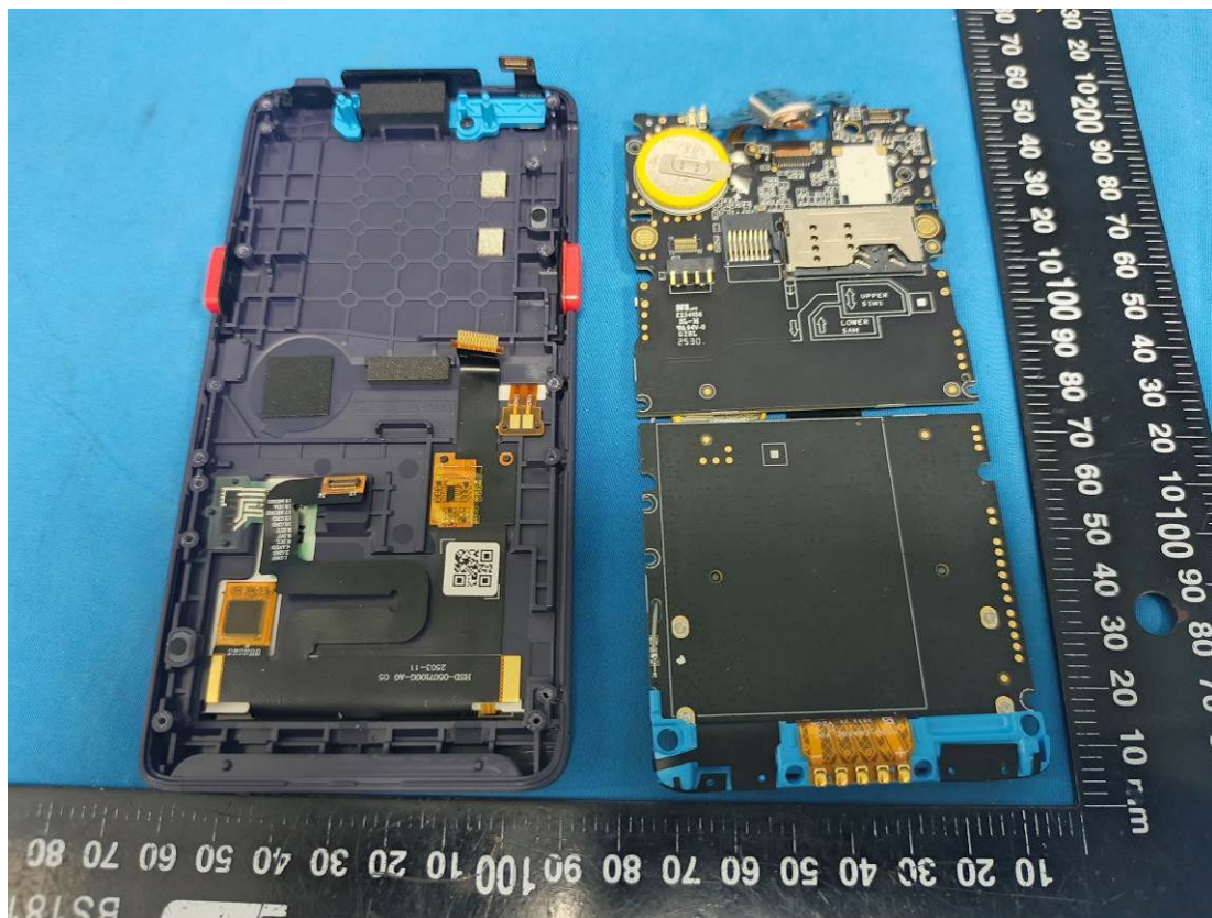
NFC Antenna
