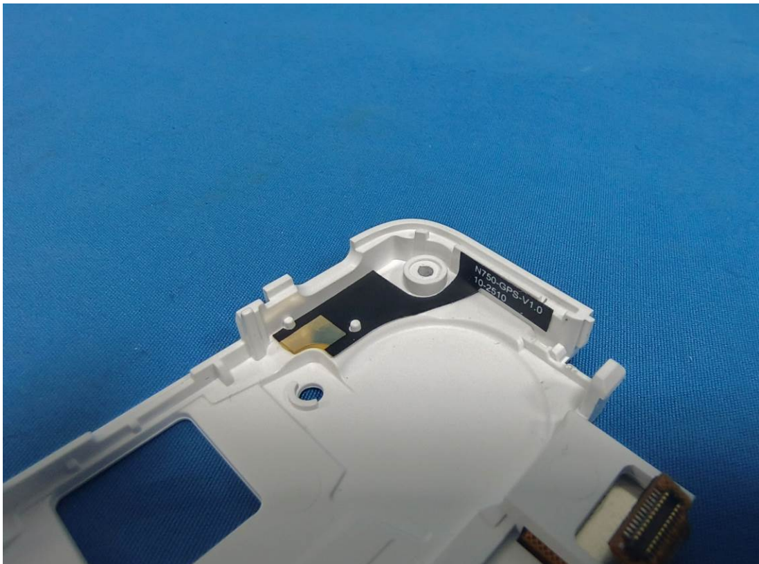
GPS Antenna
