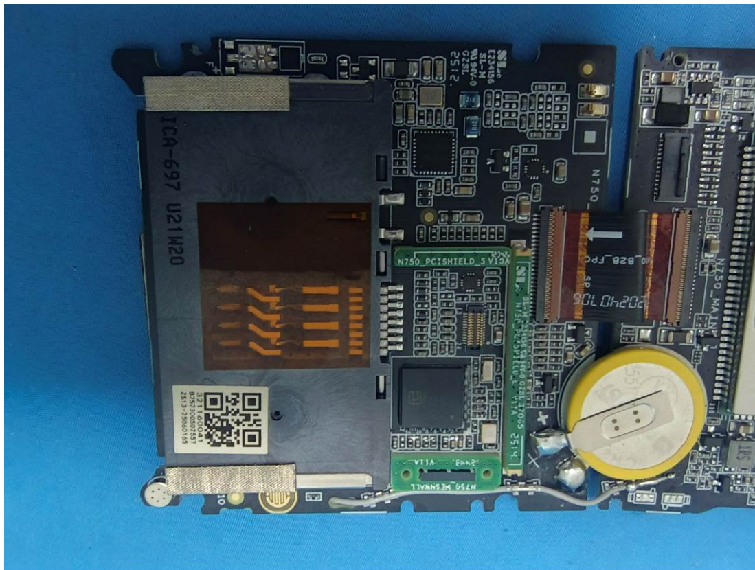
Bluetooth&Wifi Antenna
