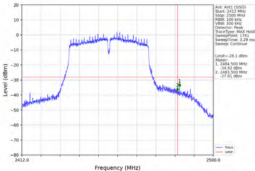
802.11n(HT40)_HCH_2452MHz_Ant1 (SISO)_NTNV
