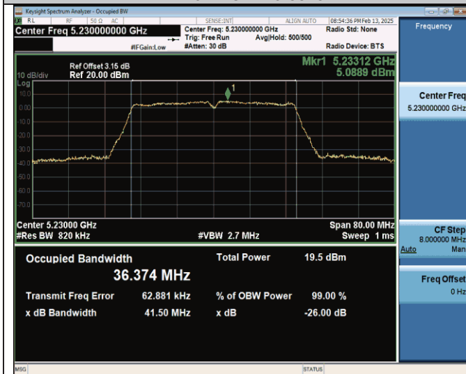
11ac40SISO-Ant0-5230
