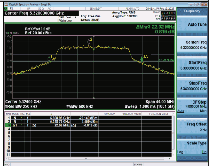
11ac20SISO-Ant0-5320
