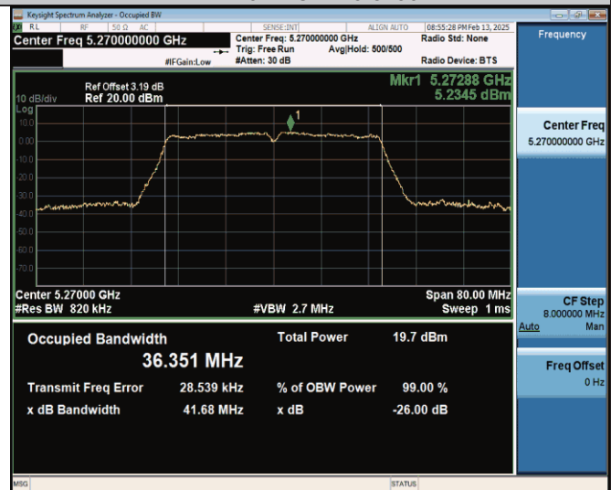
11ac40SISO-Ant0-5270
