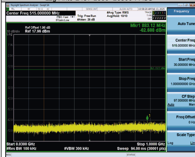
11g-Ant0-2462-30-1000-PASS
