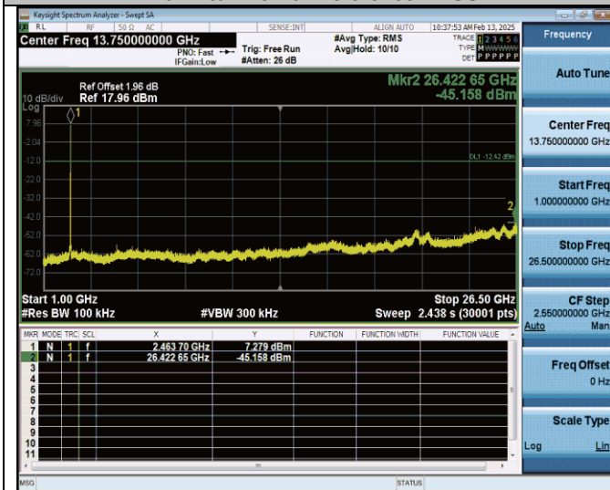
11b-Ant0-2462-1000-26500-PASS
