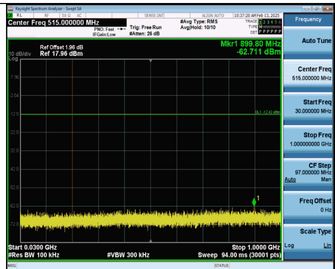
11b-Ant0-2462-30-1000-PASS
