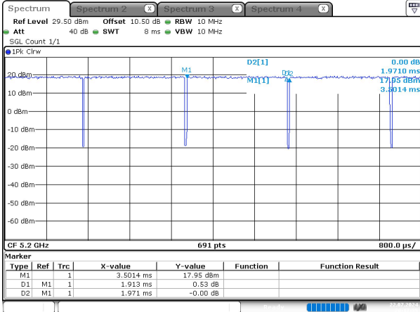
ac20_5200MHz_Chain 0
