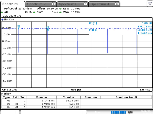
a_5200MHz_Chain 0
