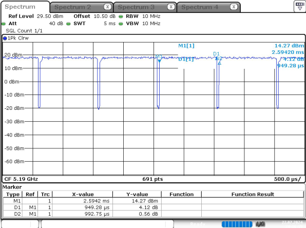
n40_5190MHz_Chain 0
