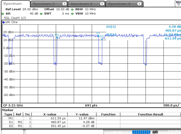
ac80_5210MHz_Chain 0
