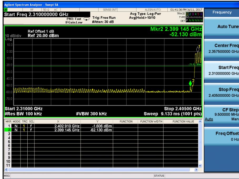
(Plot 4.5.2.1 A: Hopping Mode @ GFSK)
