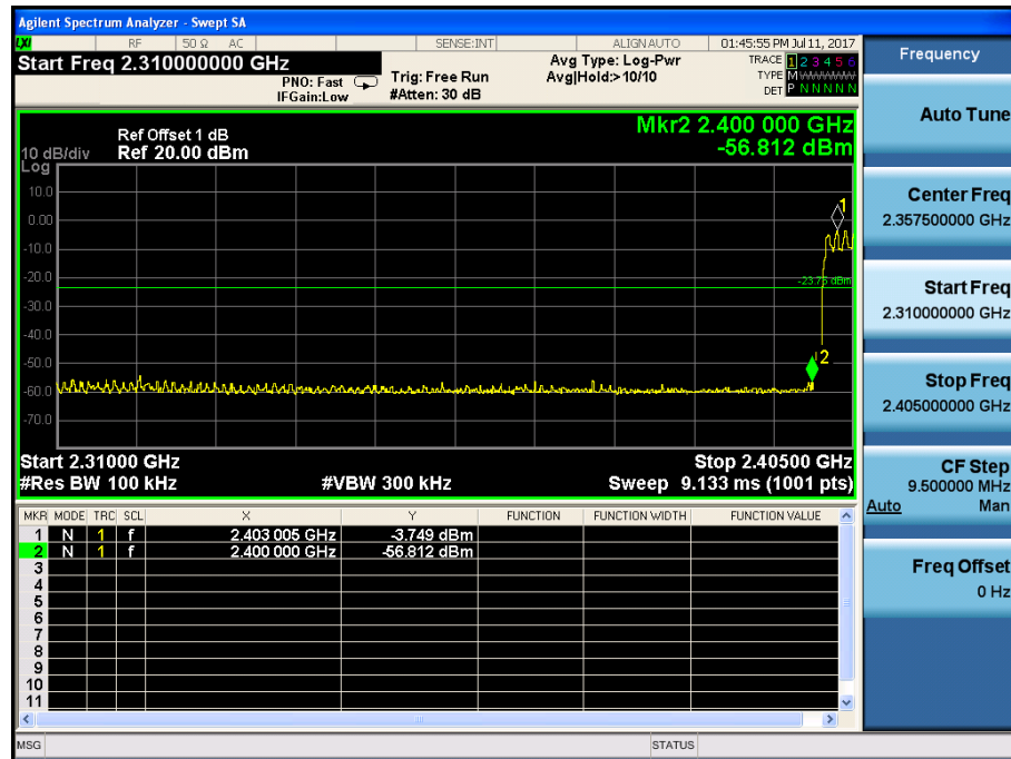
(Plot 4.5.2.2 A: Hopping Mode @ 8DPSK)
