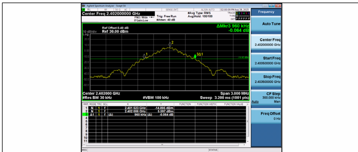
DH5-Ant1-2402
