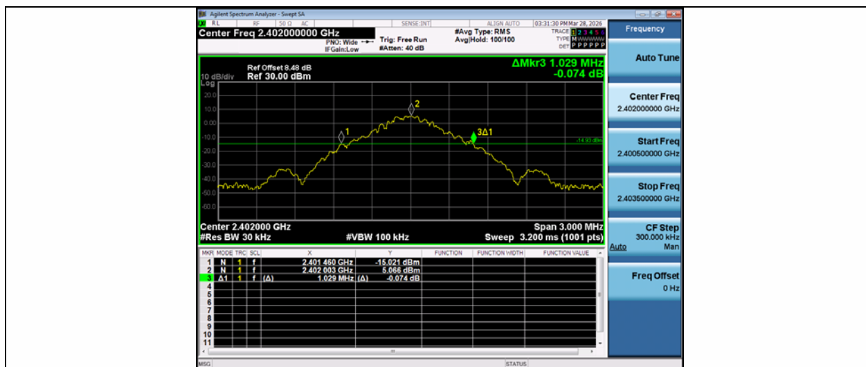
DH5-Ant1-2402
