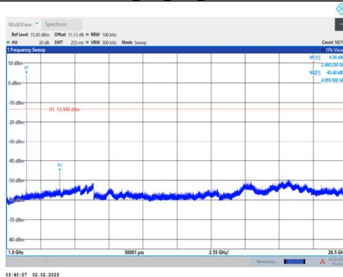
SRD2.4G_Ant2_2480_1000~26500
