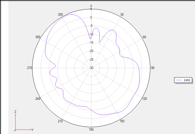
H 面
