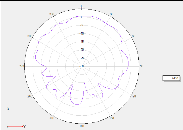
H 面
