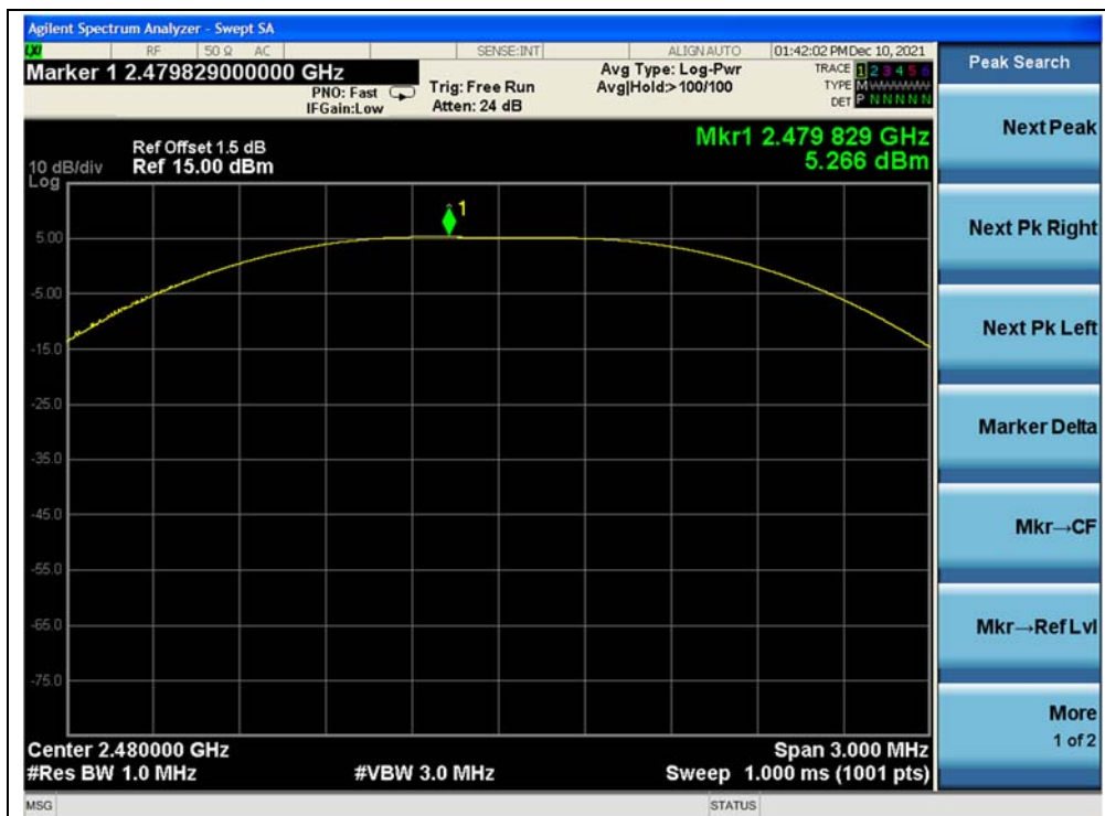
(Channel 39, 2480MHz)
