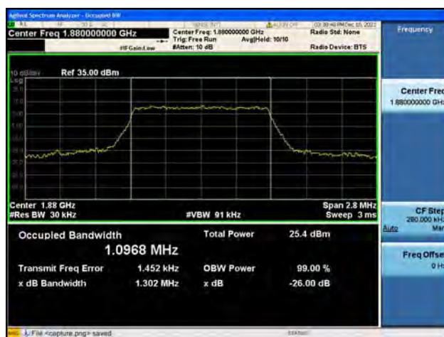
Band2 / 1.4MHz / Mid CH / 64QAM
