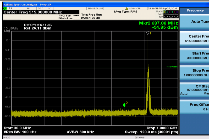
Band5-5MHz-QPSK-20425-1RB#0-30~1000MHz
