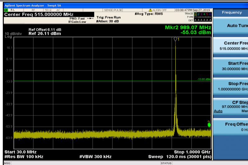
Band5-3MHz-QPSK-20415-1RB#0-30~1000MHz
