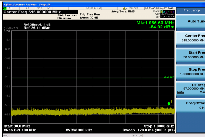
Band7-10MHz-QPSK-20800-1RB#0-30~1000MHz
