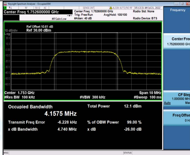
Band4-1513-5
