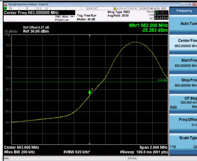
Band71-10MHz-QPSK-133172-1RB#49
