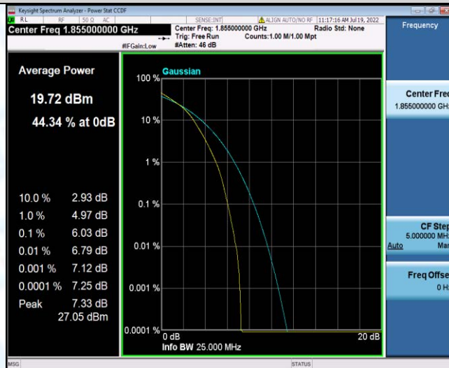
Band25-10MHz-16QAM-26365-1RB#0
