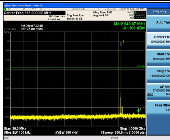
Band5-5MHz-QPSK-20425-1-0-Low-30-1000--61.11-PASS
