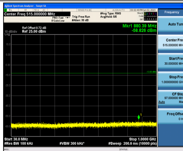
Band2-15MHz-QPSK-18900-1-0-Low-30-1000--58.83-PASS
