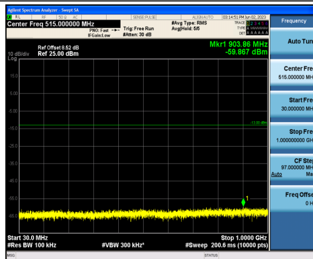
Band2-10MHz-16QAM-19150-1-0-Low-30-1000--59.87-PASS
