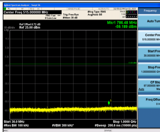
Band2-5MHz-16QAM-18900-1-0-Low-30-1000--59.19-PASS
