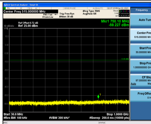
Band2-3MHz-QPSK-18900-1-0-Low-30-1000--59.23-PASS
