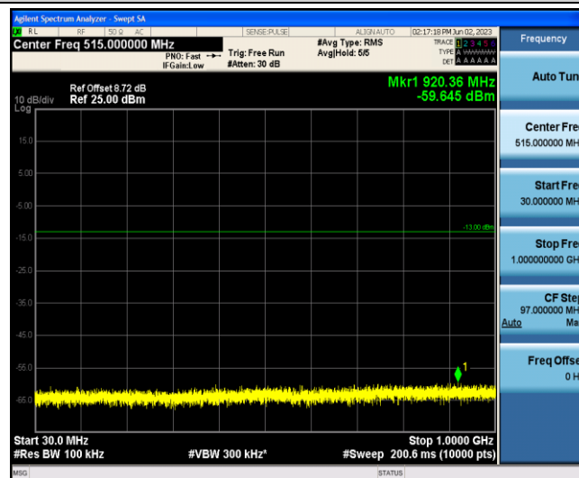
Band2-1.4MHz-16QAM-18900-1-0-Low-30-1000--59.65-PASS
