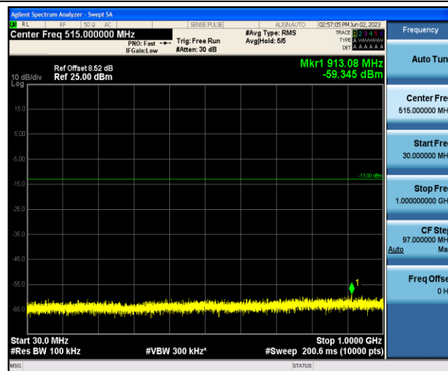
Band2-5MHz-16QAM-19175-1-0-Low-30-1000--59.35-PASS
