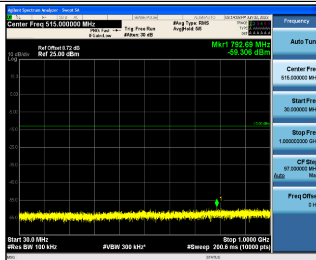
Band2-10MHz-16QAM-18900-1-0-Low-30-1000--59.31-PASS
