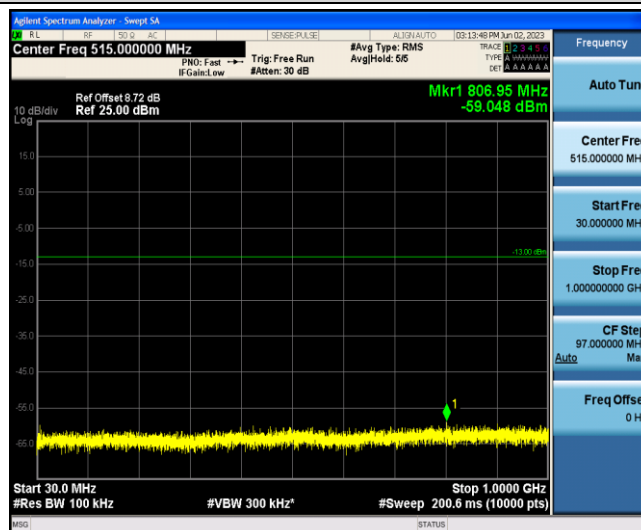
Band2-10MHz-QPSK-18900-1-0-Low-30-1000--59.05-PASS
