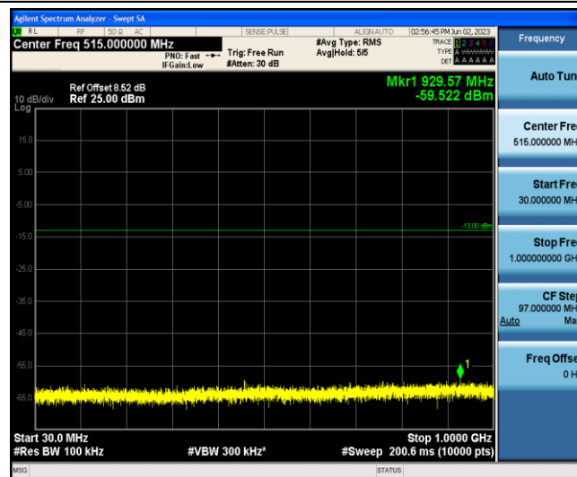
Band2-5MHz-QPSK-19175-1-0-Low-30-1000--59.52-PASS
