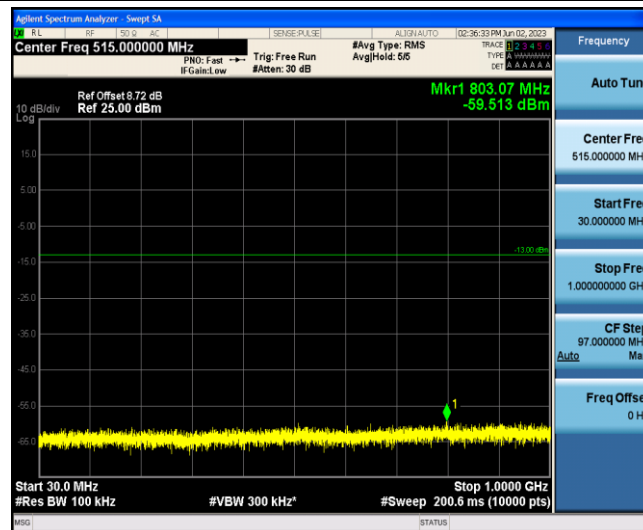
Band2-3MHz-QPSK-18615-1-0-Low-30-1000--59.51-PASS
