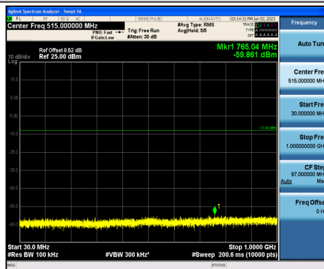
Band2-10MHz-QPSK-19150-1-0-Low-30-1000--59.86-PASS
