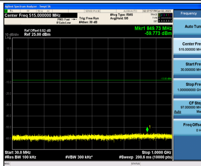
Band2-3MHz-QPSK-19185-1-0-Low-30-1000--59.77-PASS
