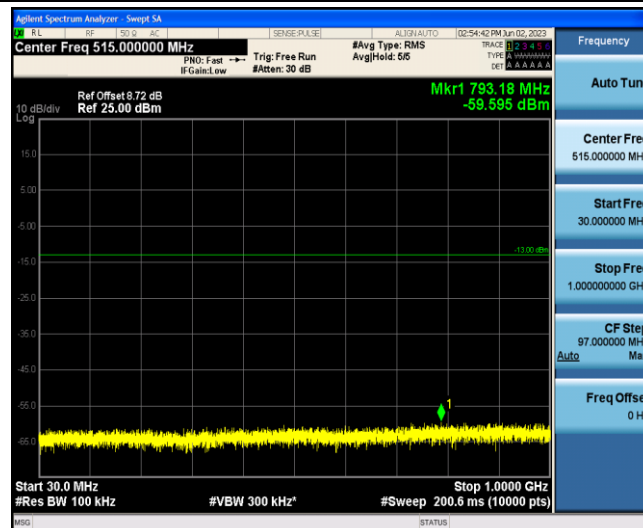
Band2-5MHz-QPSK-18900-1-0-Low-30-1000--59.6-PASS
