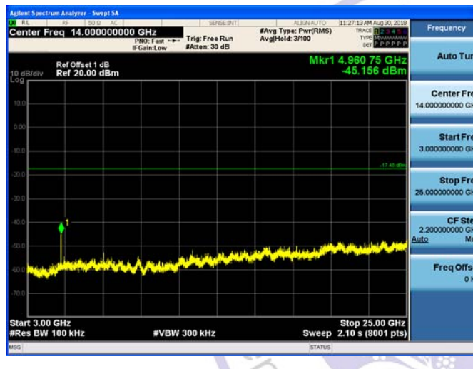
3GHz-25GHz
