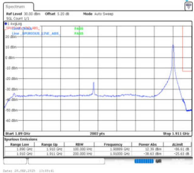
Band2-20MHz-QPSK-19100-1RB#99-PASS
