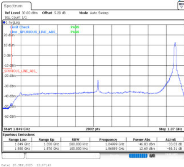
Band2-20MHz-16QAM-18700-1RB#99-PASS
