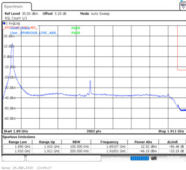
Band2-20MHz-QPSK-19100-1RB#0-PASS
