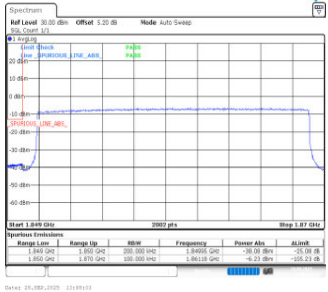
Band2-20MHz-16QAM-18700-100RB#0-PASS
