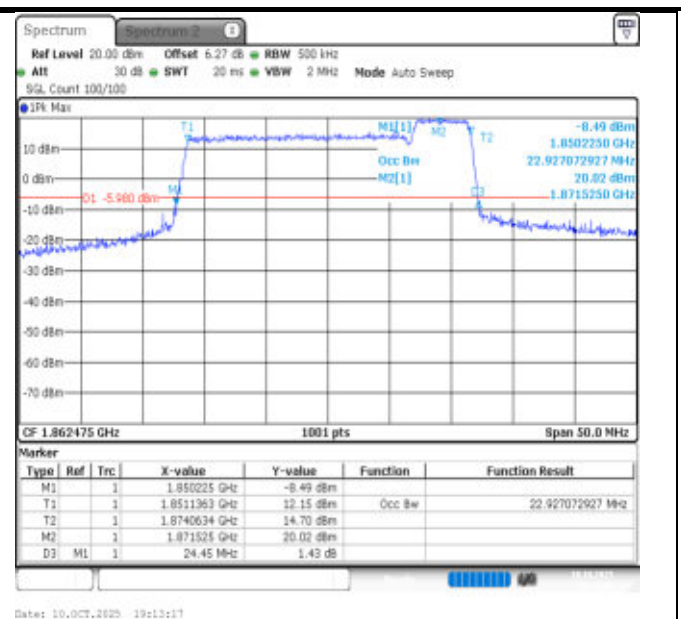
2-2-20MHz-5MHz-16QAM-16QAM-18700-18817-100RB#0-25RB#0-PASS
