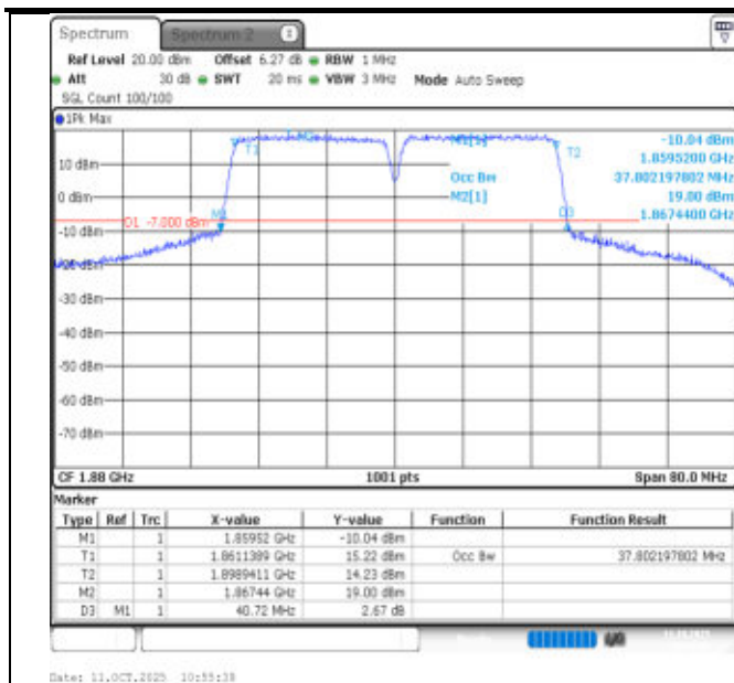
2-2-20MHz-20MHz-QPSK-QPSK-18801-18999-100RB#0-100RB#0-PASS
