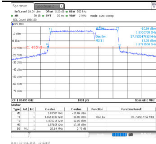
2-2-20MHz-10MHz-QPSK-QPSK-18700-18844-100RB#0-50RB#0-PASS
