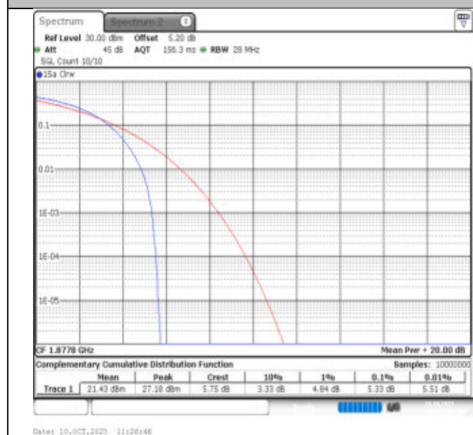
2-2-10MHz-20MHz-QPSK-QPSK-18806-18950-50RB#0- 100RB#0-PASS
