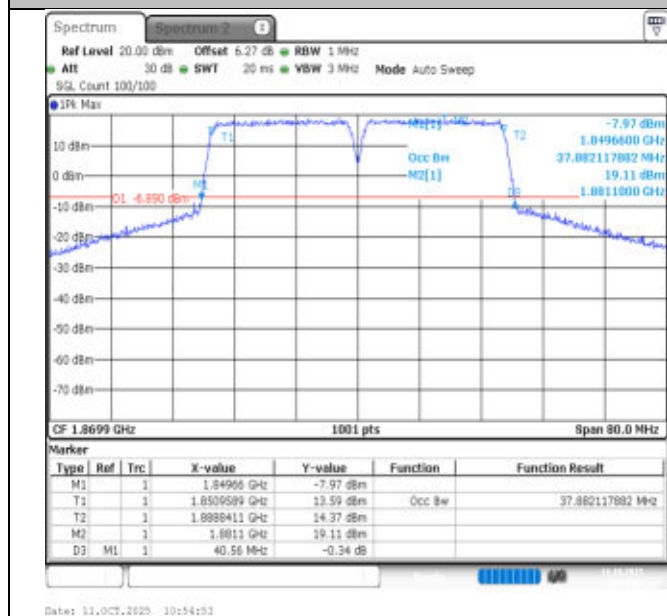
2-2-20MHz-20MHz-QPSK-QPSK-18700-18898-100RB#0-100RB#0-PASS
