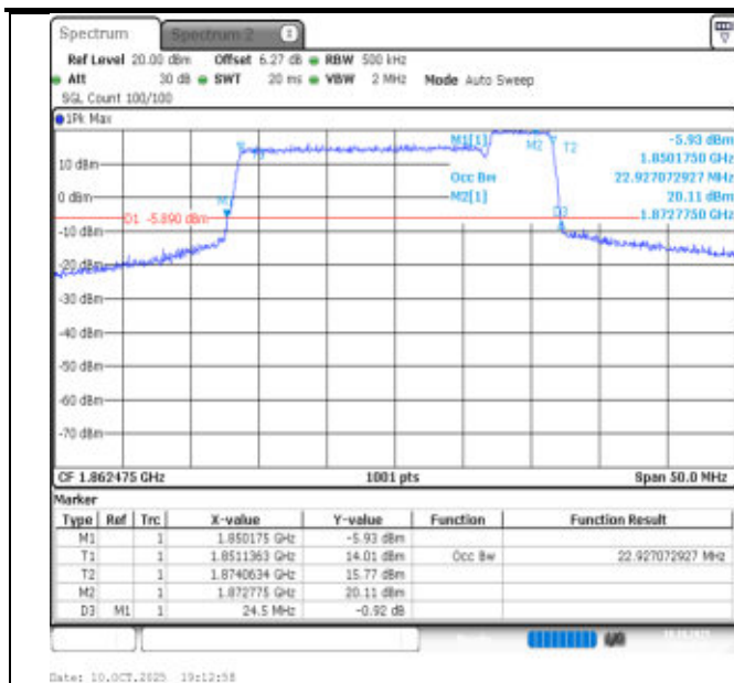
2-2-20MHz-5MHz-QPSK-QPSK-18700-18817-100RB#0-25RB#0-PASS
