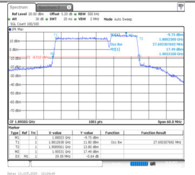
2-2-20MHz-10MHz-16QAM-16QAM-19001-19145-100RB#0-50RB#0-PASS
