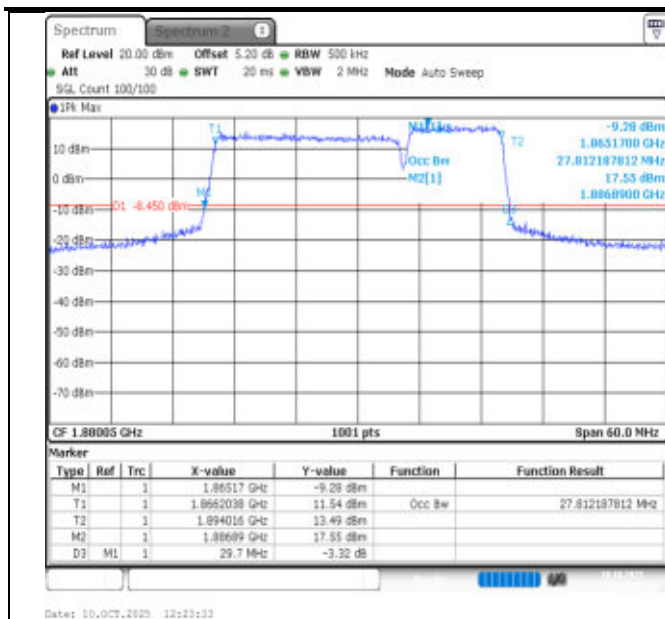
2-2-20MHz-10MHz-QPSK-QPSK-18851-18995-100RB#0-50RB#0-PASS
