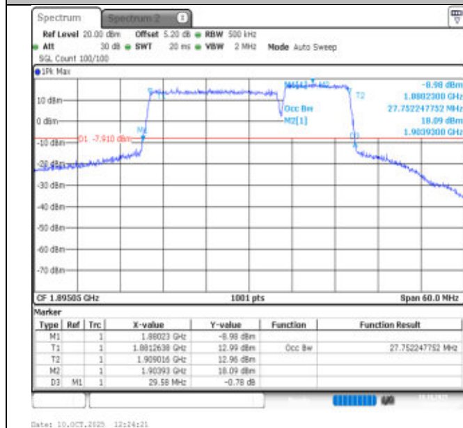
2-2-20MHz-10MHz-QPSK-QPSK-19001-19145-100RB#0-50RB#0-PASS
