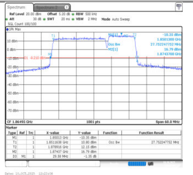
2-2-20MHz-10MHz-16QAM-16QAM-18700-18844-100RB#0-50RB#0-PASS
