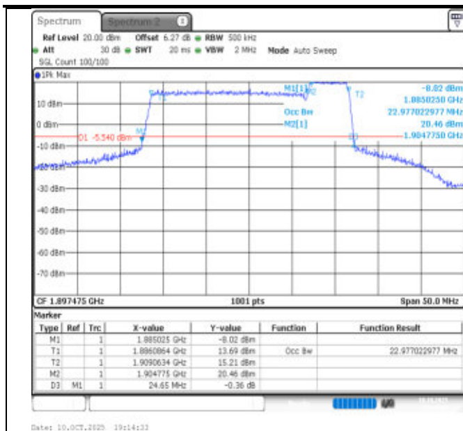
2-2-20MHz-5MHz-QPSK-QPSK-19050-19167-100RB#0-25RB#0-PASS
