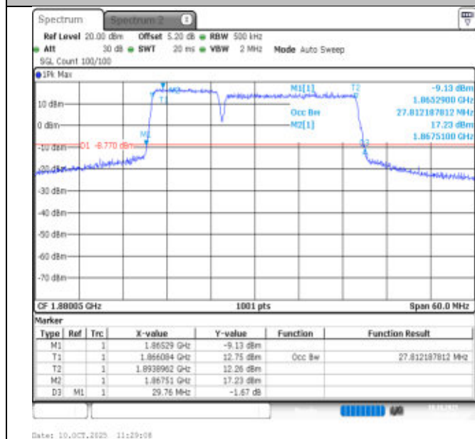
2-2-10MHz-20MHz-QPSK-QPSK-18806-18950-50RB#0-100RB#0-PASS
