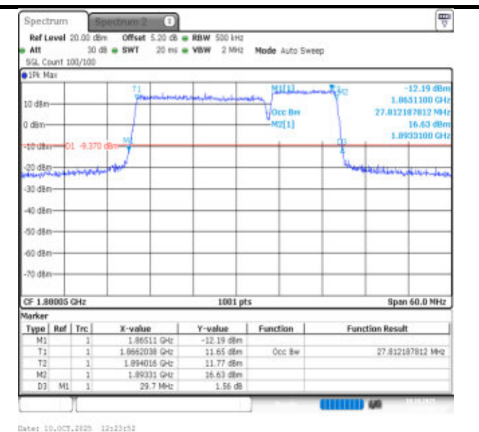
2-2-20MHz-10MHz-16QAM-16QAM-18851-18995-100RB#0-50RB#0-PASS
