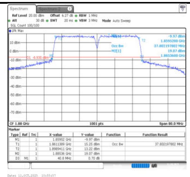
2-2-20MHz-20MHz-16QAM-16QAM-18801-18999-100RB#0-100RB#0-PASS
