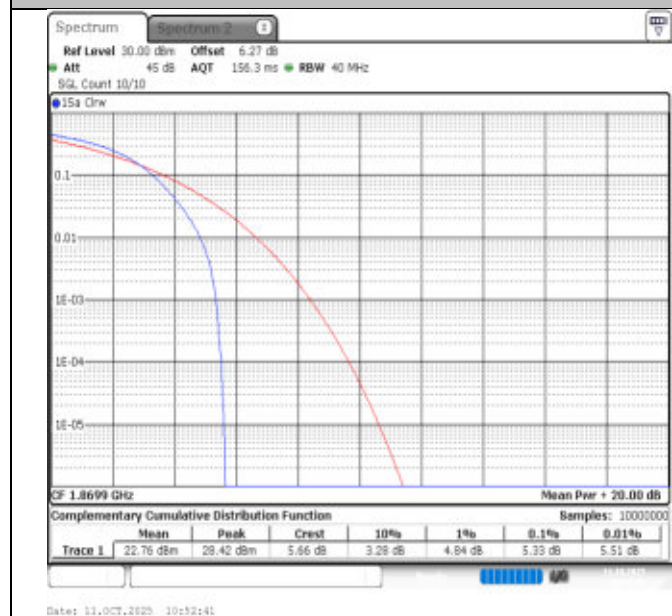
2-2-20MHz-20MHz-QPSK-QPSK-18700-18898-100RB#0-100RB#0-PASS
