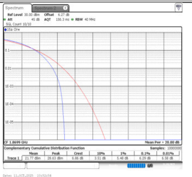
2-2-20MHz-20MHz-16QAM-16QAM-18700-18898-100RB#0-100RB#0-PASS
