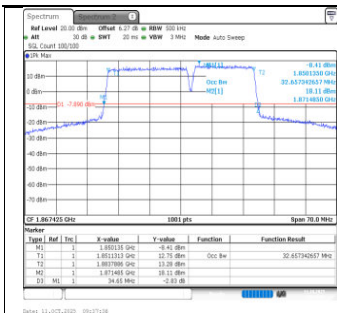
2-2-20MHz-15MHz-QPSK-QPSK-18700-18871-100RB#0-75RB#0-PASS
