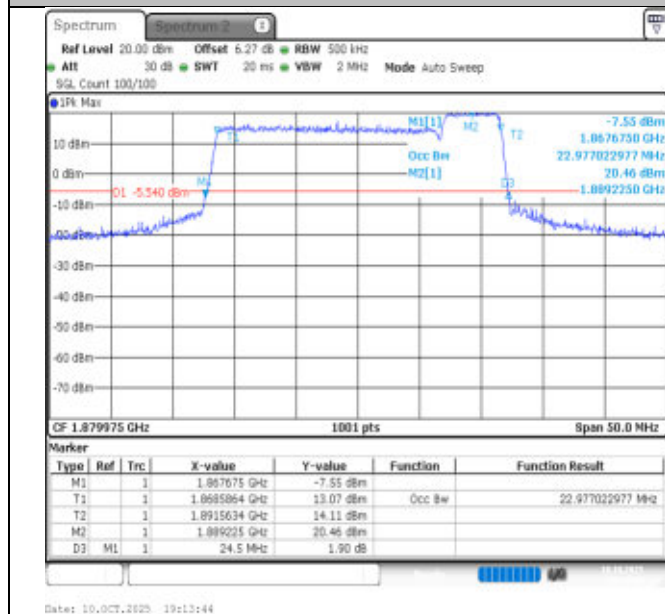
2-2-20MHz-5MHz-QPSK-QPSK-18875-18992-100RB#0-25RB#0-PASS
