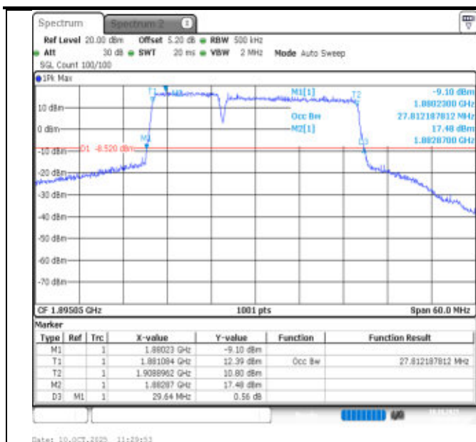
2-2-10MHz-20MHz-QPSK-QPSK-18956-19100-50RB#0-100RB#0-PASS
