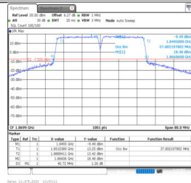
2-2-20MHz-20MHz-16QAM-16QAM-18700-18898-100RB#0-100RB#0-PASS
