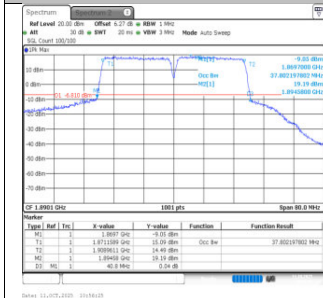
2-2-20MHz-20MHz-QPSK-QPSK-18902-19100-100RB#0-100RB#0-PASS
