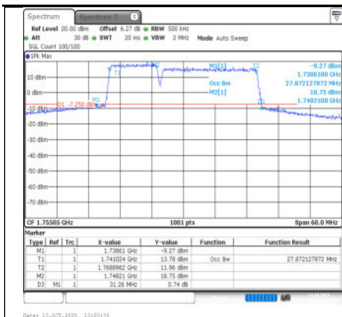
66-66-10MHz-20MHz-QPSK-QPSK-132328-132472-50RB#0-100RB#0-PASS
