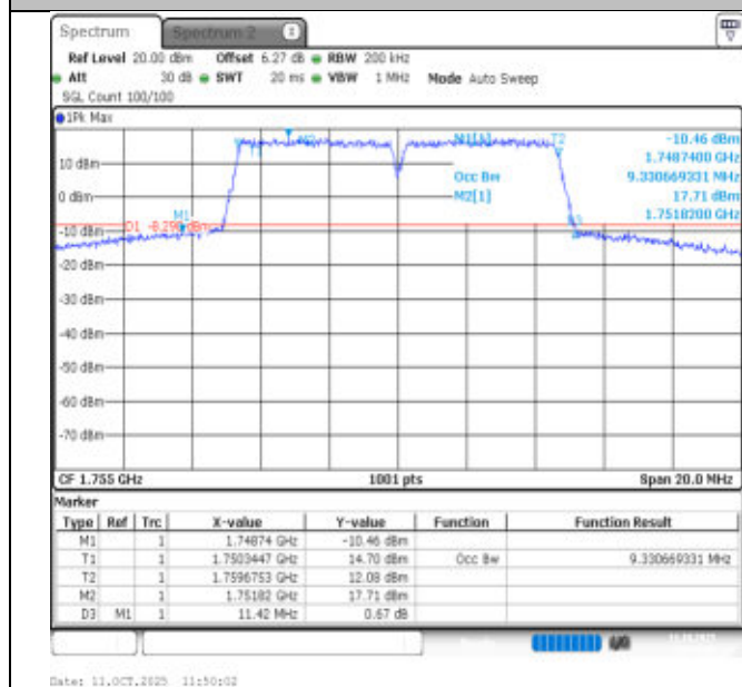
66-66-5MHz-5MHz-QPSK-QPSK-132398-132446-25RB#0-25RB#0-PASS
