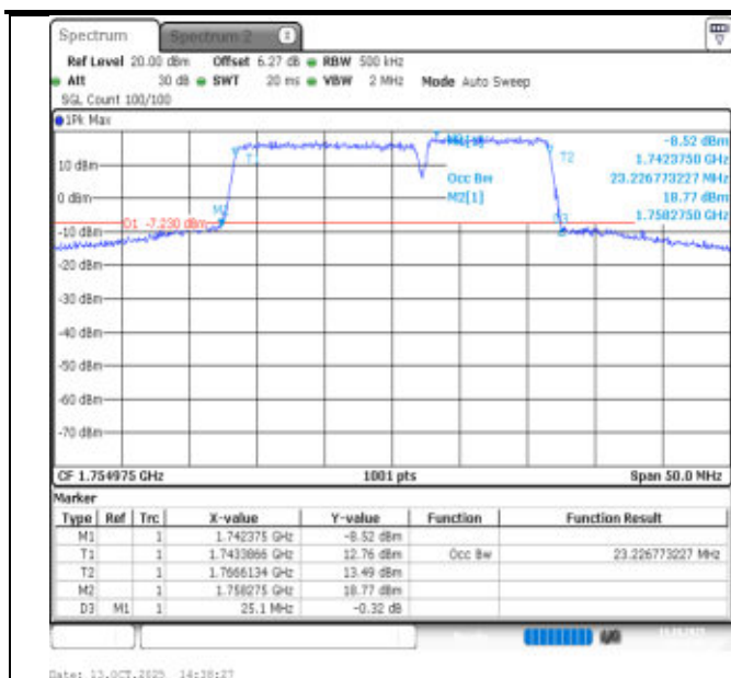
66-66-15MHz-10MHz-QPSK-QPSK-132373-132493-75RB#0-50RB#0-PASS
