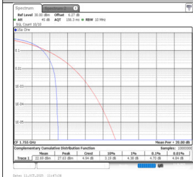
66-66-5MHz-5MHz-QPSK-QPSK-132398-132446-25RB#0-25RB#0-PASS
