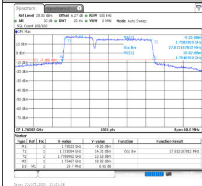
66-66-10MHz-20MHz-QPSK-QPSK-132428-132572-50RB#0-100RB#0-PASS
