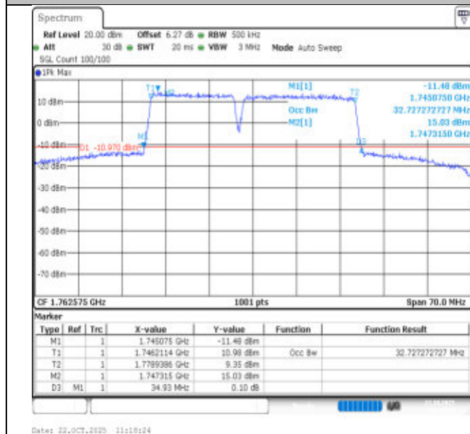
66-66-15MHz-20MHz-QPSK-QPSK-132401-132572-75RB#0-100RB#0-PASS
