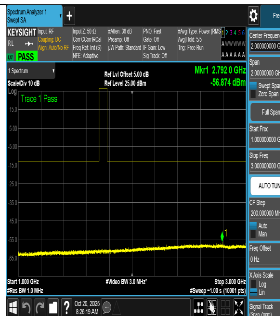
NTNV-n66-PC3-15-5-L-DFT-QPSK- Inner_1RB_Left-1000-3000-PASS
