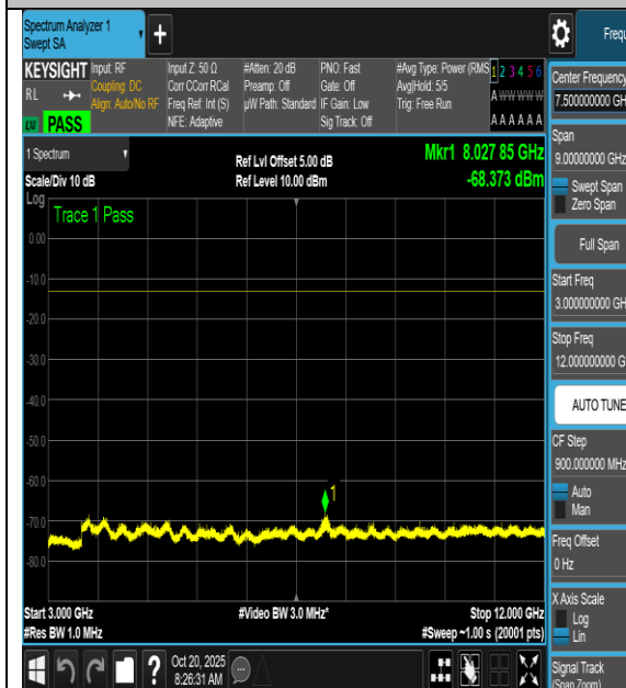
NTNV-n66-PC3-15-5-L-DFT-QPSK- Inner_1RB_Left-3000-12000-PASS
