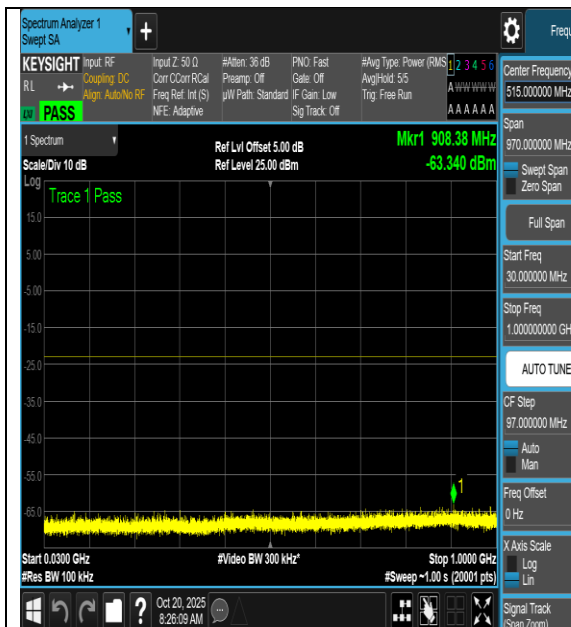
NTNV-n66-PC3-15-5-L-DFT-QPSK- Inner_1RB_Left-30-1000-PASS
