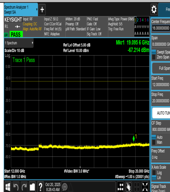
NTNV-n66-PC3-15-5-L-DFT-QPSK- Inner_1RB_Left-12000-20000-PASS
