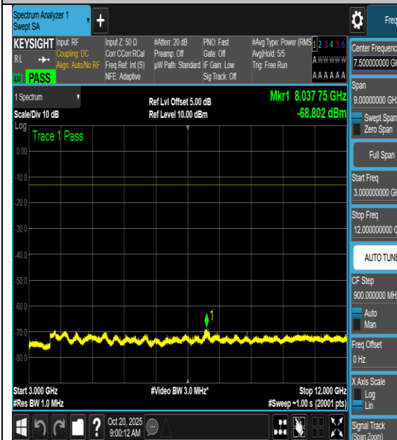
NTNV-n66-PC3-15-5-L-CP-QPSK- Inner_1RB_Left-3000-12000-PASS
