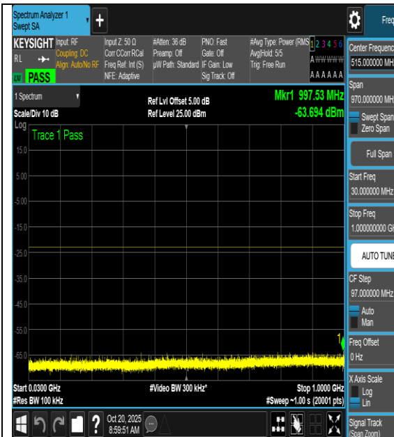
NTNV-n66-PC3-15-5-L-CP-QPSK- Inner_1RB_Left-30-1000-PASS
