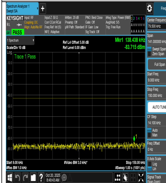
NTNV-n66-PC3-15-5-L-CP-QPSK- Edge_1RB_Left-0.009-0.15-PASS
