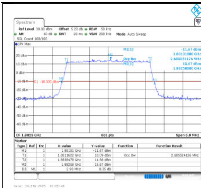
Band25-3MHz-QPSK-26365-15RB#0-PASS
