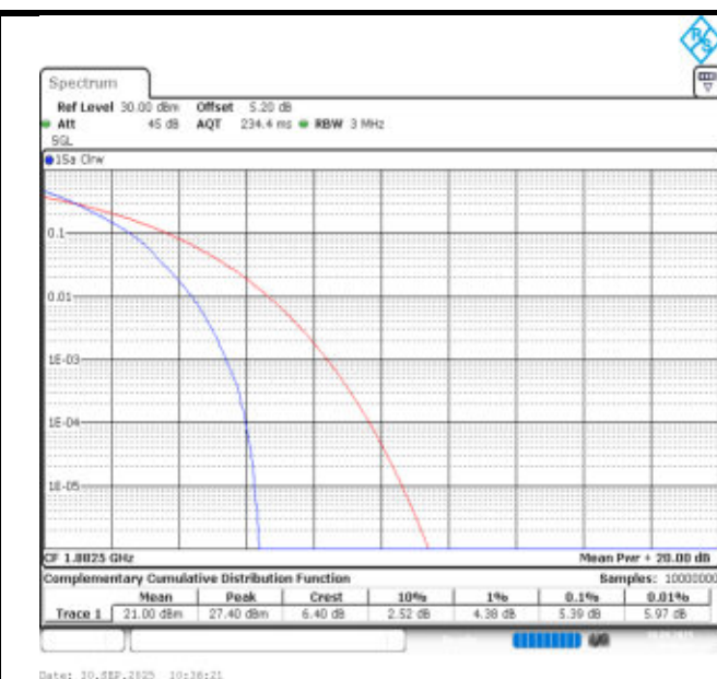
Band25-3MHz-QPSK-26365-15RB#0-PASS
