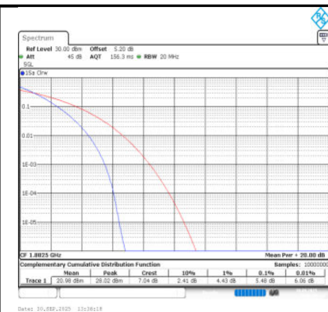
Band25-20MHz-QPSK-26365-100RB#0-PASS
