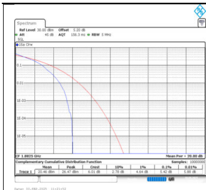
Band25-5MHz-QPSK-26365-1RB#0-PASS
