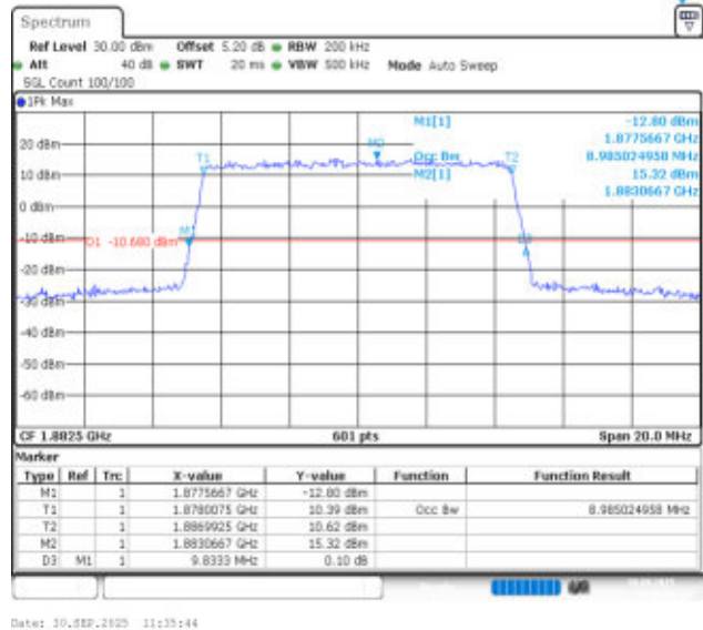
Band25-10MHz-16QAM-26365-50RB#0-PASS
