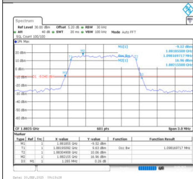
Band25-1.4MHz-QPSK-26365-6RB#0-PASS
