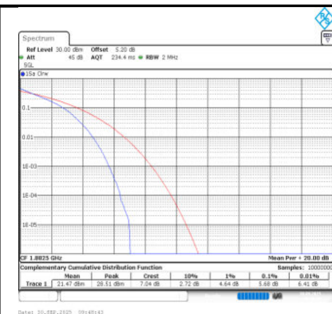
Band25-1.4MHz-QPSK-26365-6RB#0-PASS
