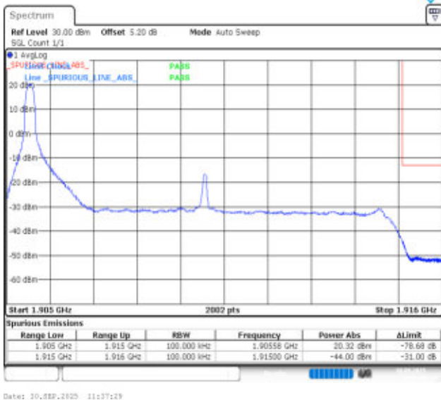
Band25-10MHz-QPSK-26640-1RB#0-PASS
