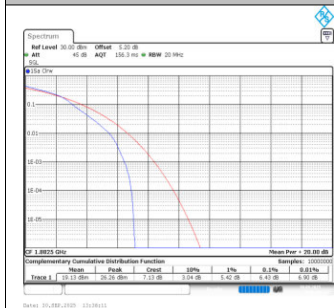
Band25-20MHz-16QAM-26365-1RB#0-PASS
