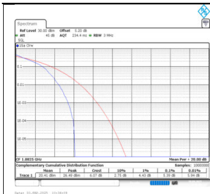
Band25-3MHz-QPSK-26365-1RB#0-PASS
