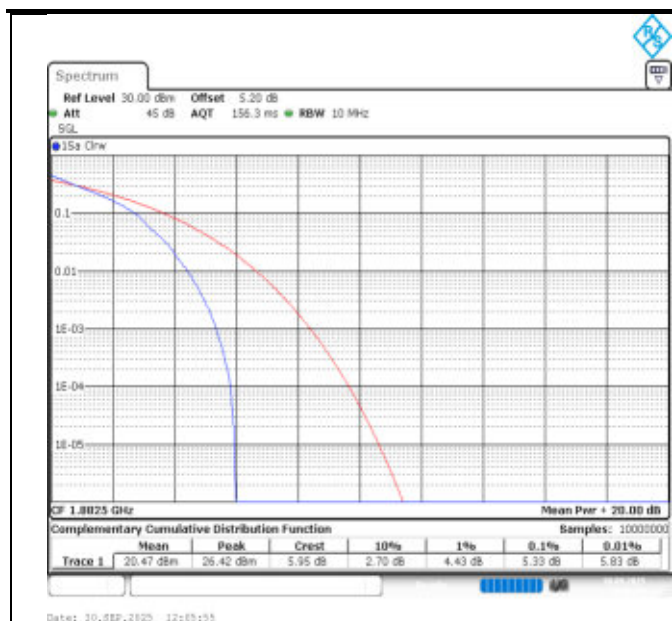
Band25-10MHz-QPSK-26365-1RB#0-PASS
