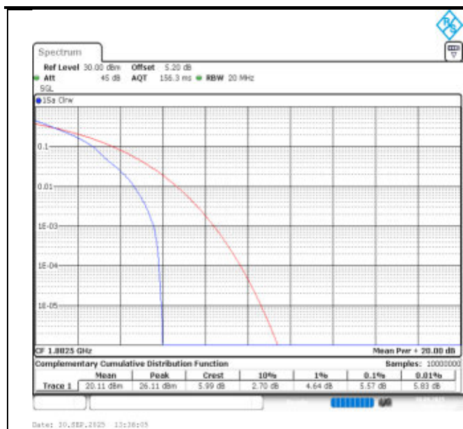
Band25-20MHz-QPSK-26365-1RB#0-PASS
