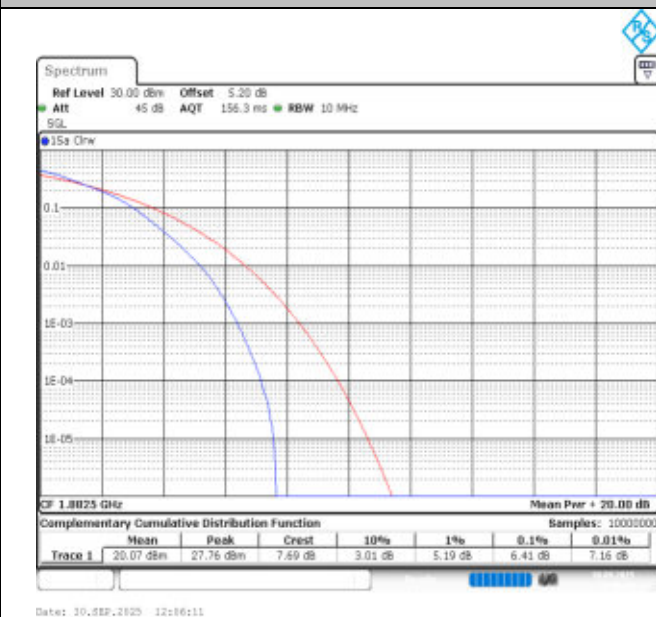
Band25-10MHz-16QAM-26365-50RB#0-PASS
