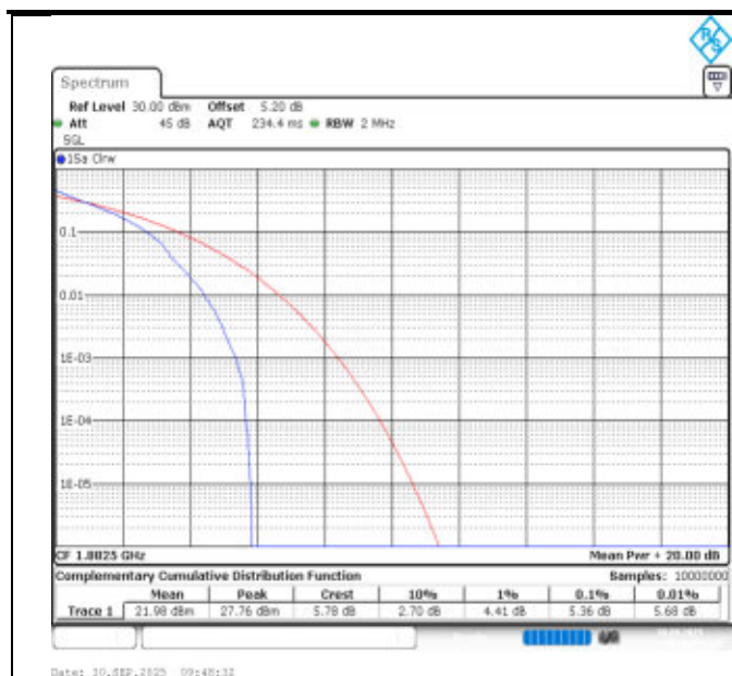
Band25-1.4MHz-QPSK-26365-1RB#0-PASS
