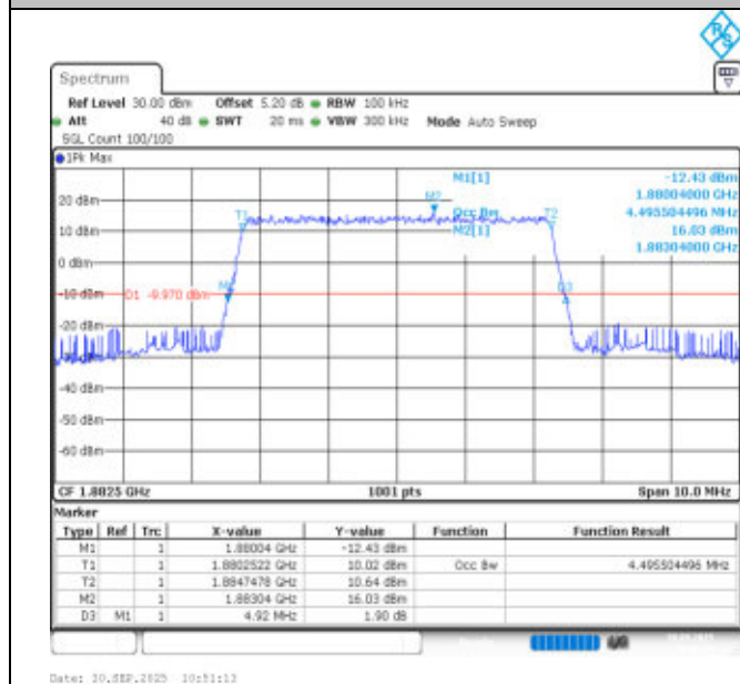
Band25-5MHz-QPSK-26365-25RB#0-PASS
