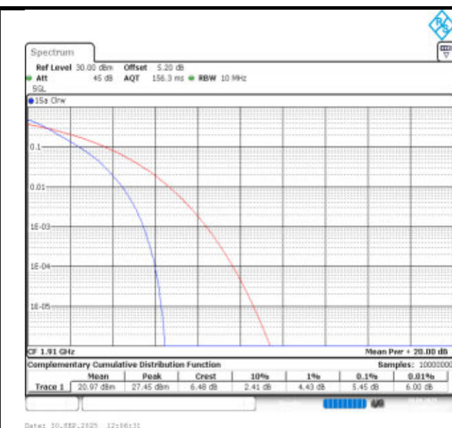
Band25-10MHz-QPSK-26640-50RB#0-PASS
