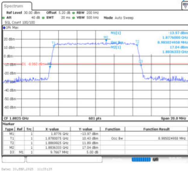
Band25-10MHz-QPSK-26365-50RB#0-PASS
