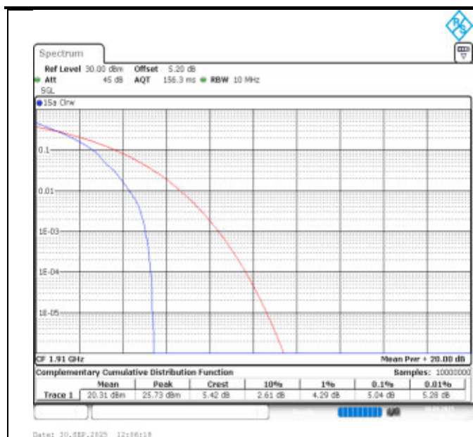
Band25-10MHz-QPSK-26640-1RB#0-PASS
