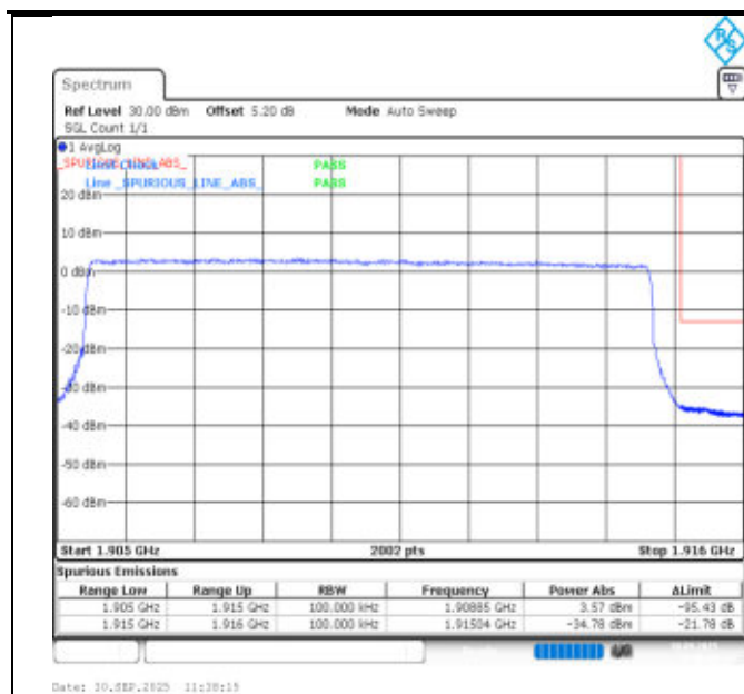
Band25-10MHz-QPSK-26640-50RB#0-PASS
