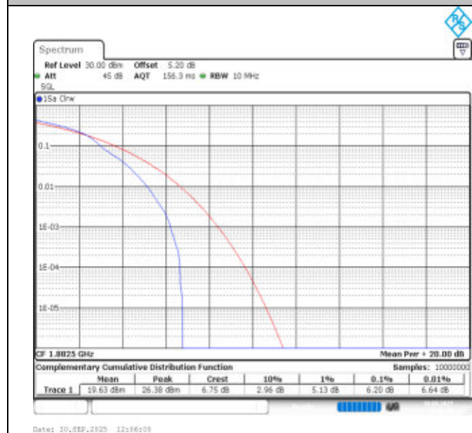
Band25-10MHz-16QAM-26365-1RB#0-PASS
