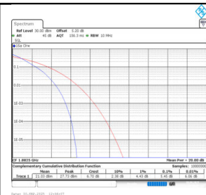
Band25-10MHz-QPSK-26365-50RB#0-PASS
