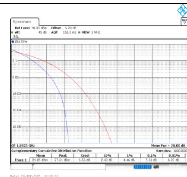
Band25-5MHz-QPSK-26365-25RB#0-PASS
