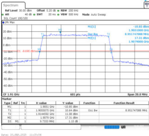
Band25-10MHz-QPSK-26640-50RB#0-PASS
