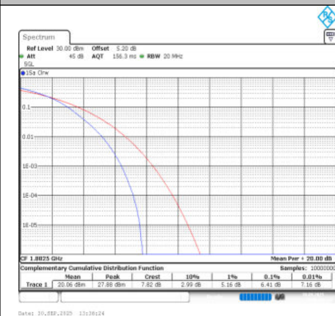
Band25-20MHz-16QAM-26365-100RB#0-PASS
