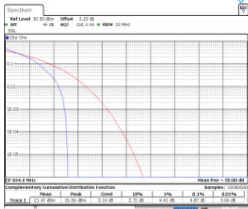
Band26(824-849)-10MHz-QPSK-26990-1RB#0-PASS
