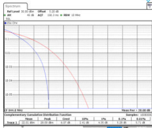
Band26(824-849)-10MHz-QPSK-26990-50RB#0-PASS
