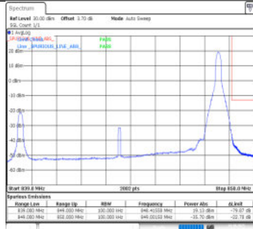
Band26(824-849)-10MHz-QPSK-26990-50RB#0-PASS
