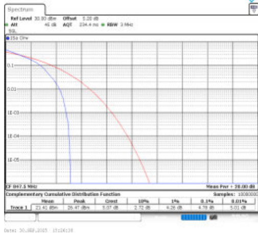
Band26(824-849)-3MHz-QPSK-27025-1RB#0-PASS
