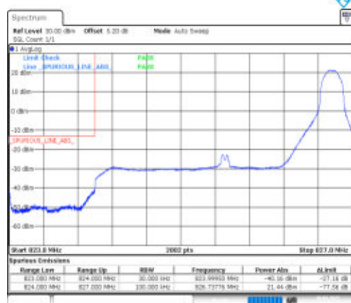
Band26(824-849)-3MHz-QPSK-26805-1RB#14-PASS
