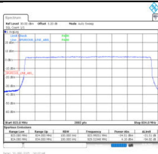
Band26(824-849)-10MHz-QPSK-26840-50RB#0-PASS
