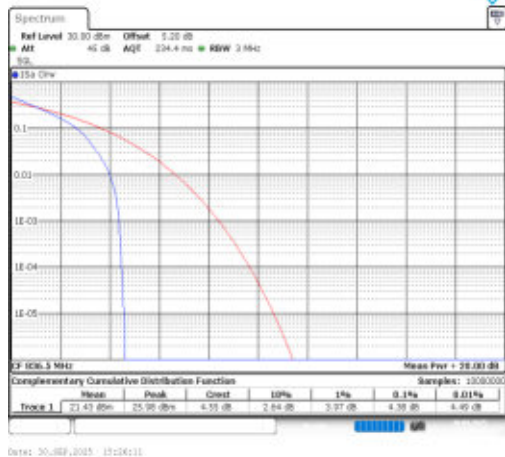
Band26(824-849)-3MHz-QPSK-26915-1RB#0-PASS
