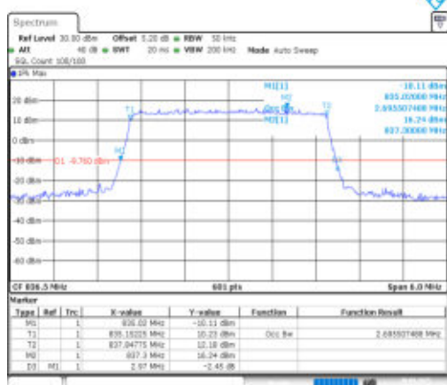
Band26(824-849)-3MHz-QPSK-26915-15RB#0-PASS
