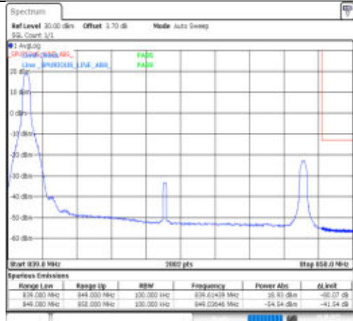
Band26(824-849)-10MHz-QPSK-26990-1RB#49-PASS
