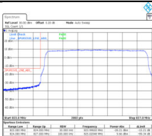
Band26(824-849)-3MHz-QPSK-26805-15RB#0-PASS
