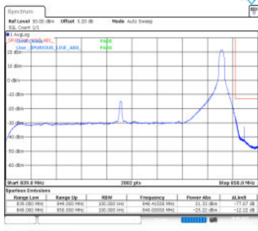
Band26(824-849)-10MHz-QPSK-26990-1RB#49-PASS
