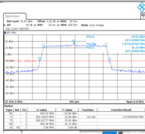
Band26(824-849)-3MHz-QPSK-26805-15RB#0-PASS
