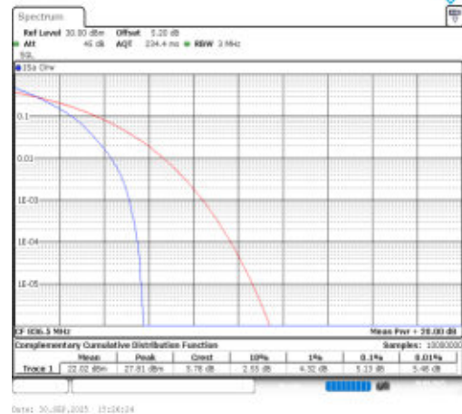
Band26(824-849)-3MHz-QPSK-26915-15RB#0-PASS
