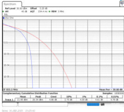
Band26(824-849)-3MHz-QPSK-26805-1RB#0-PASS
