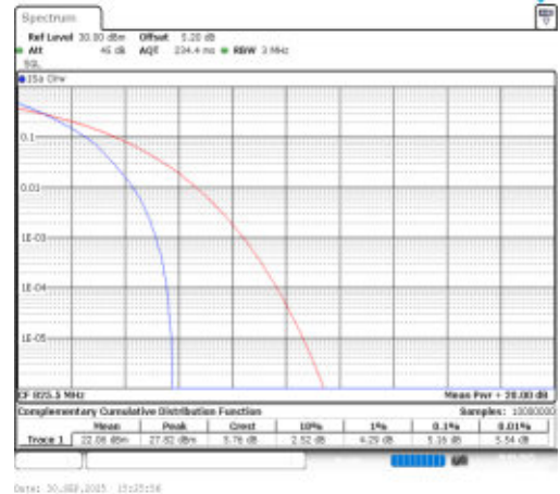
Band26(824-849)-3MHz-QPSK-26805-15RB#0-PASS
