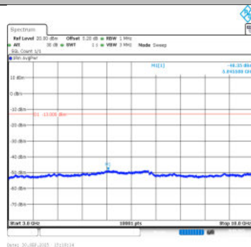
Band26(824-849)-3MHz-QPSK-27025-1RB#0- 3000~10000-PASS
