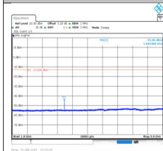
Band26(824-849)-3MHz-QPSK-27025-1RB#0- 1000~3000-PASS
