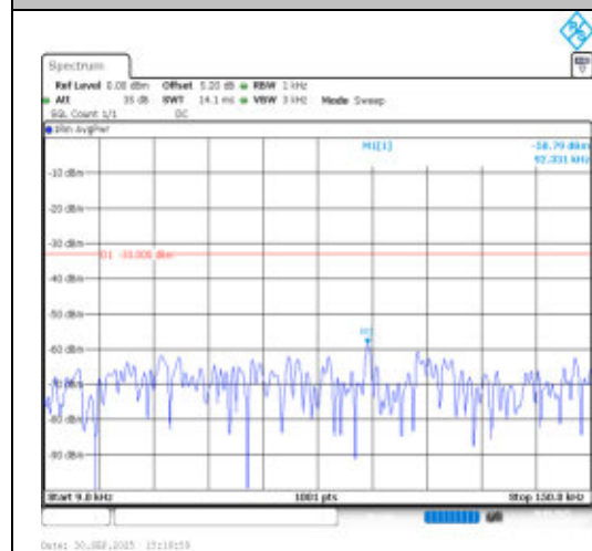
Band26(824-849)-3MHz-QPSK-27025-1RB#14- 0.009~0.15-PASS
