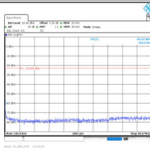
Band26(824-849)-3MHz-QPSK-27025-1RB#14- 0.15~30-PASS
