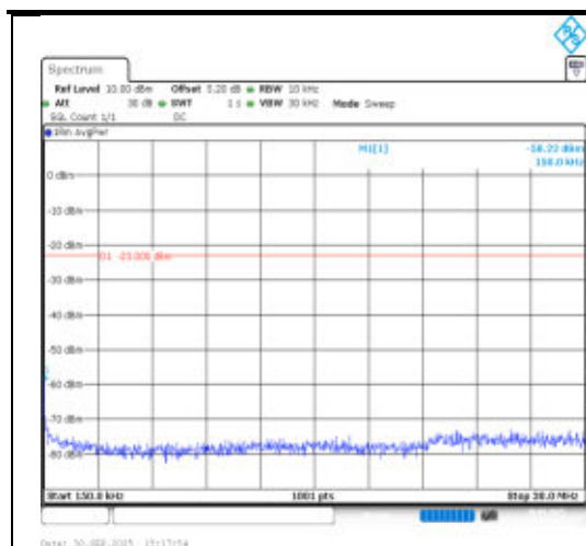
Band26(824-849)-3MHz-QPSK-27025-1RB#0- 0.15~30-PASS
