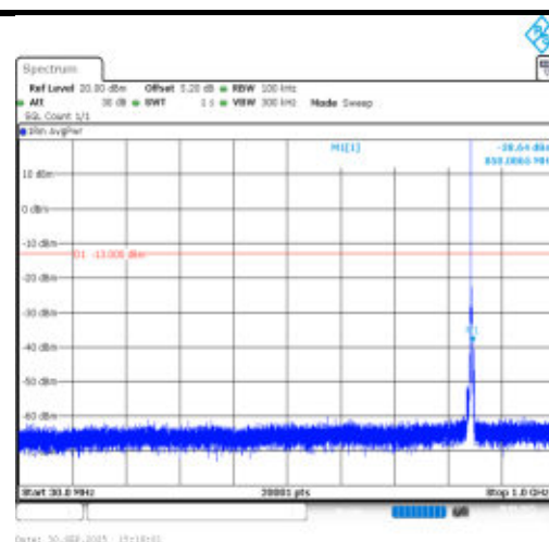
Band26(824-849)-3MHz-QPSK-27025-1RB#0- 30~1000-PASS
