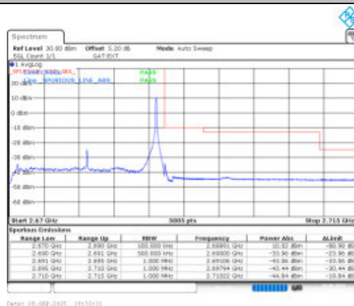
Band41-20MHz-QPSK-41490-1RB#99-PASS
