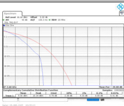
Band41-20MHz-QPSK-41490-1RB#0-PASS
