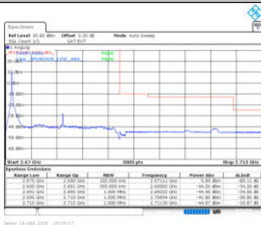
Band41-20MHz-QPSK-41490-1RB#0-PASS
