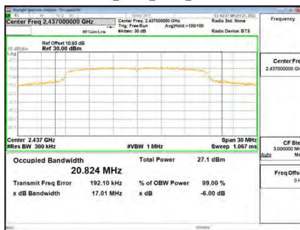
802.11n_20MHz_Chain1_2437MHz
