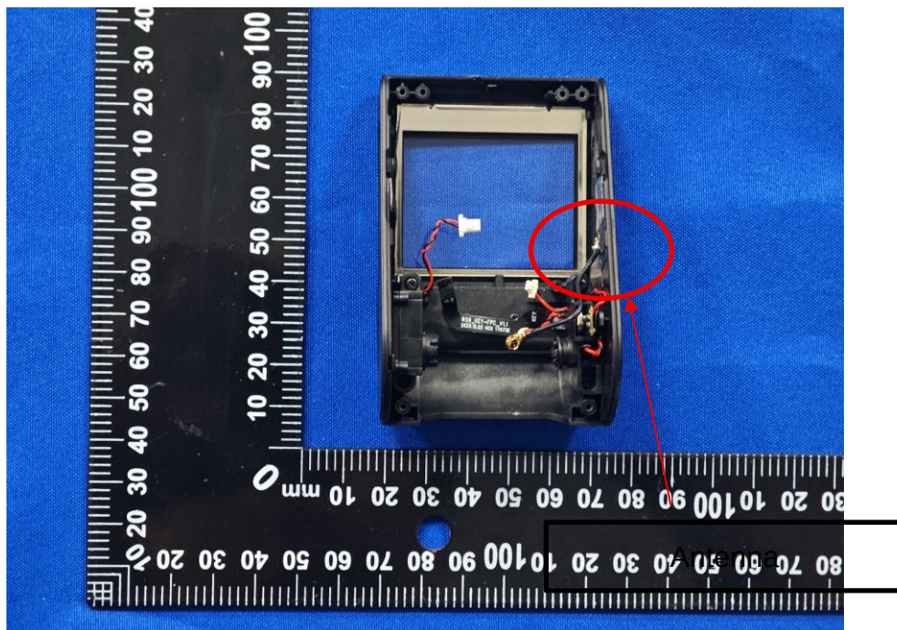
EUT Photo 20
