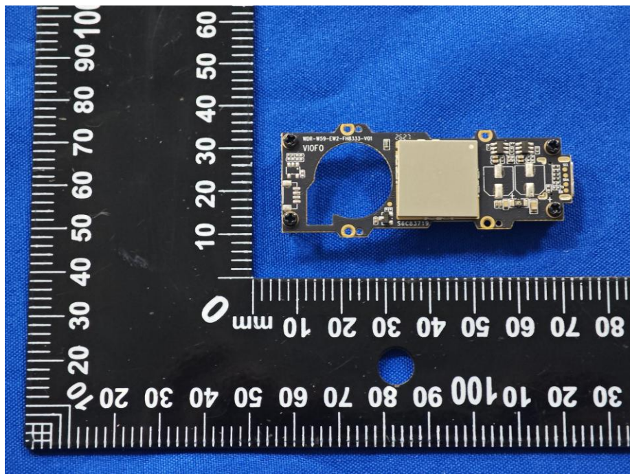
EUT Photo 30
