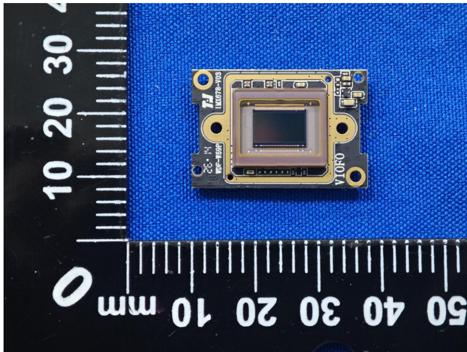
EUT Photo 19
