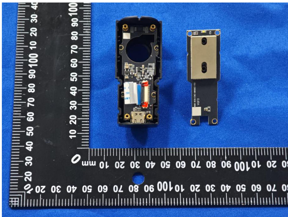
EUT Photo 24
