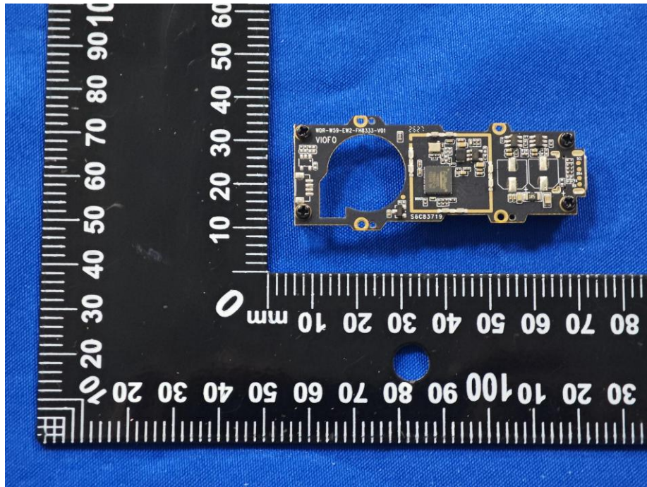
EUT Photo 31
