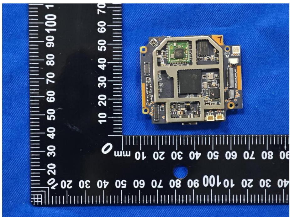
EUT Photo 13
