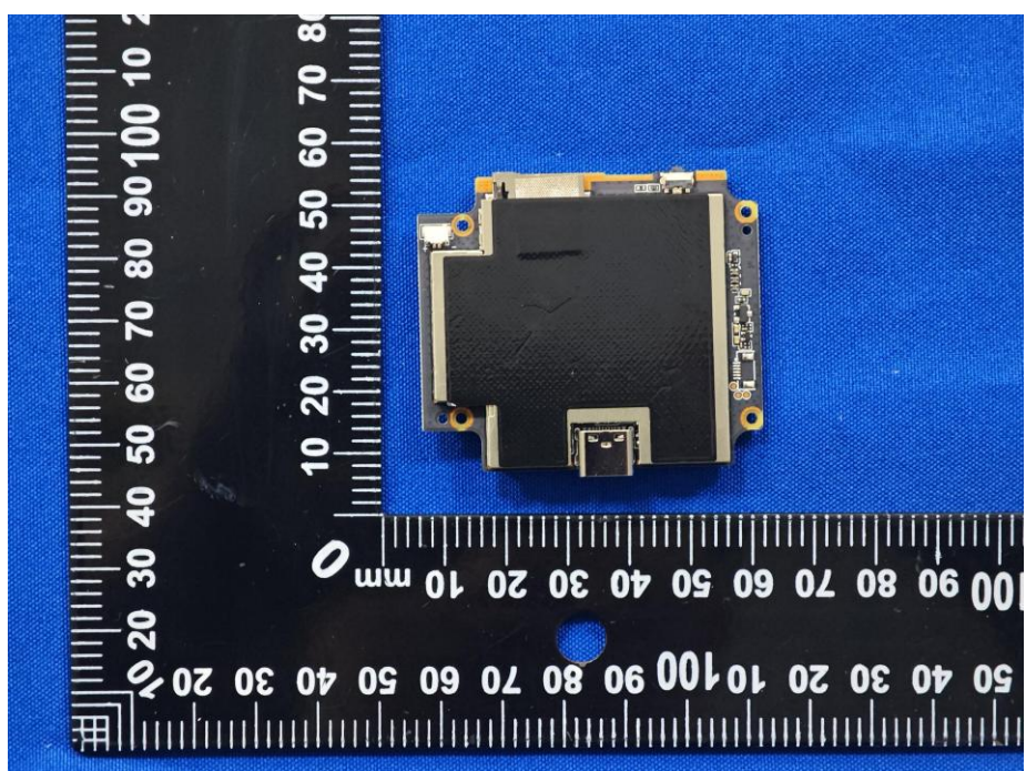
EUT Photo 14
