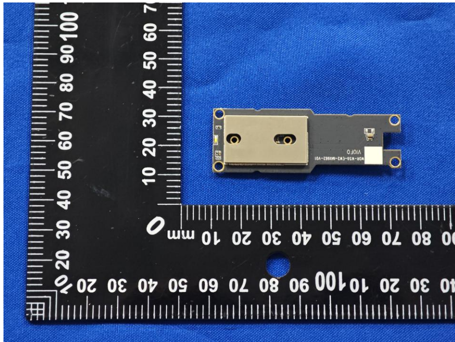
EUT Photo 25
