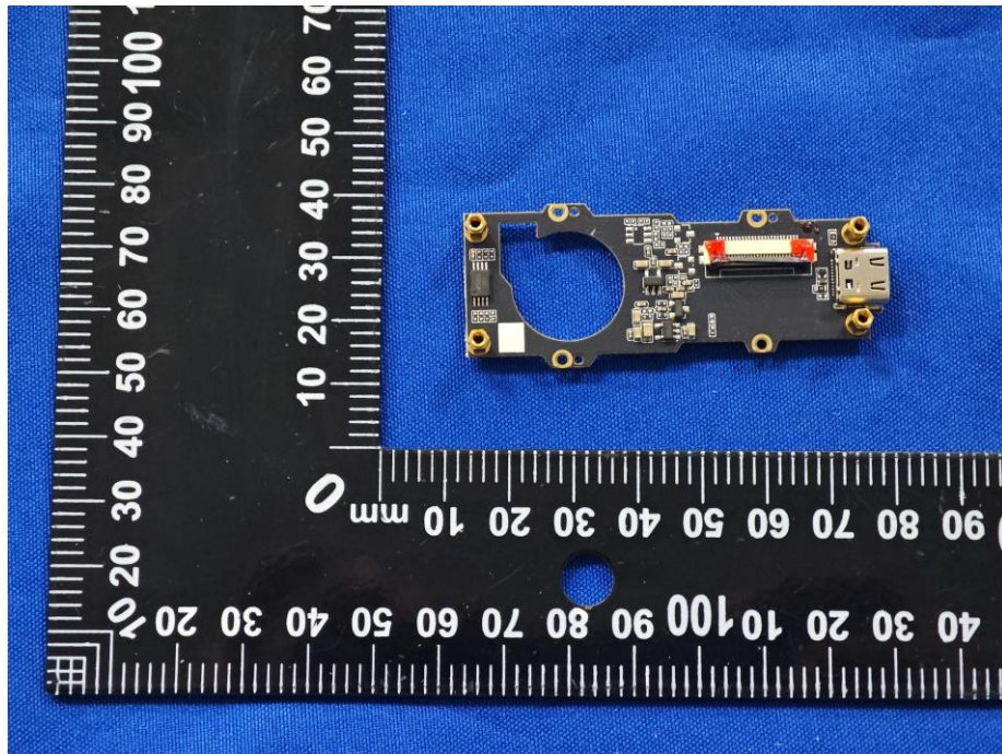
EUT Photo 29
