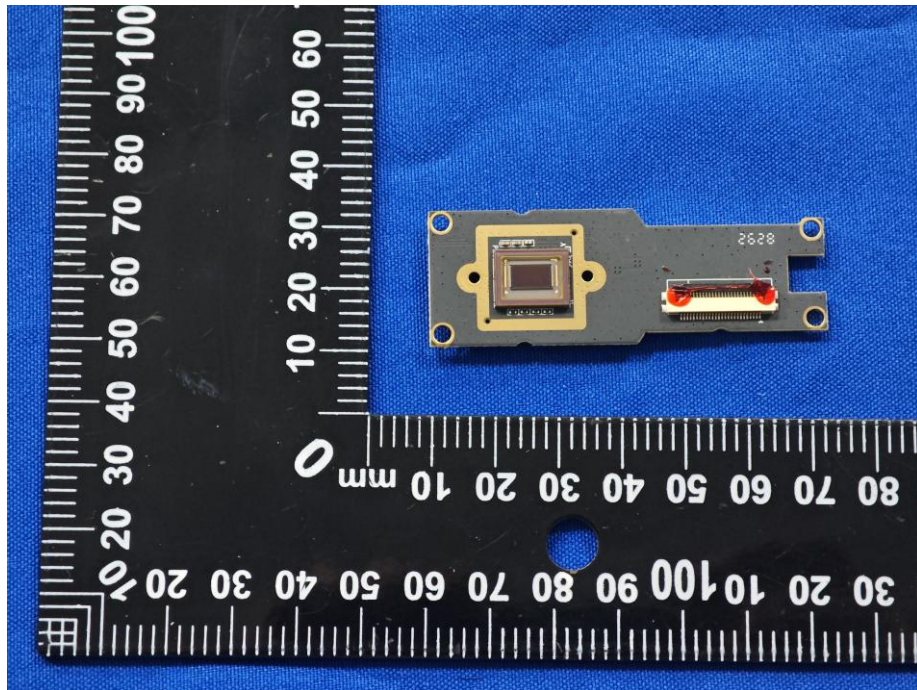
EUT Photo 27
