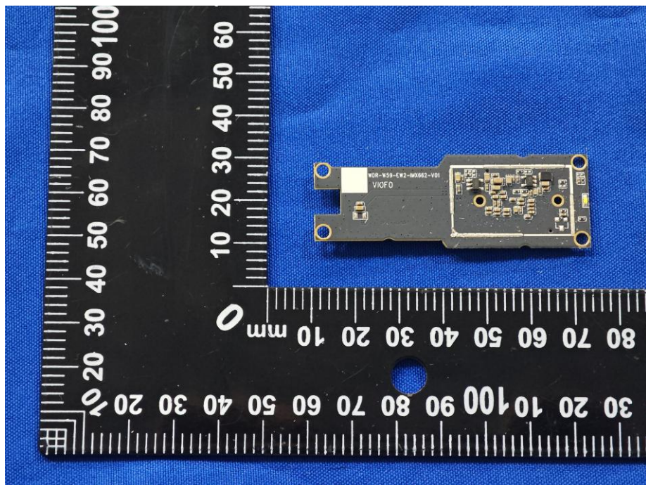
EUT Photo 26
