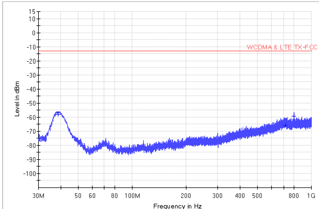
WCDMA & LTE TX 30M-1GdBm
