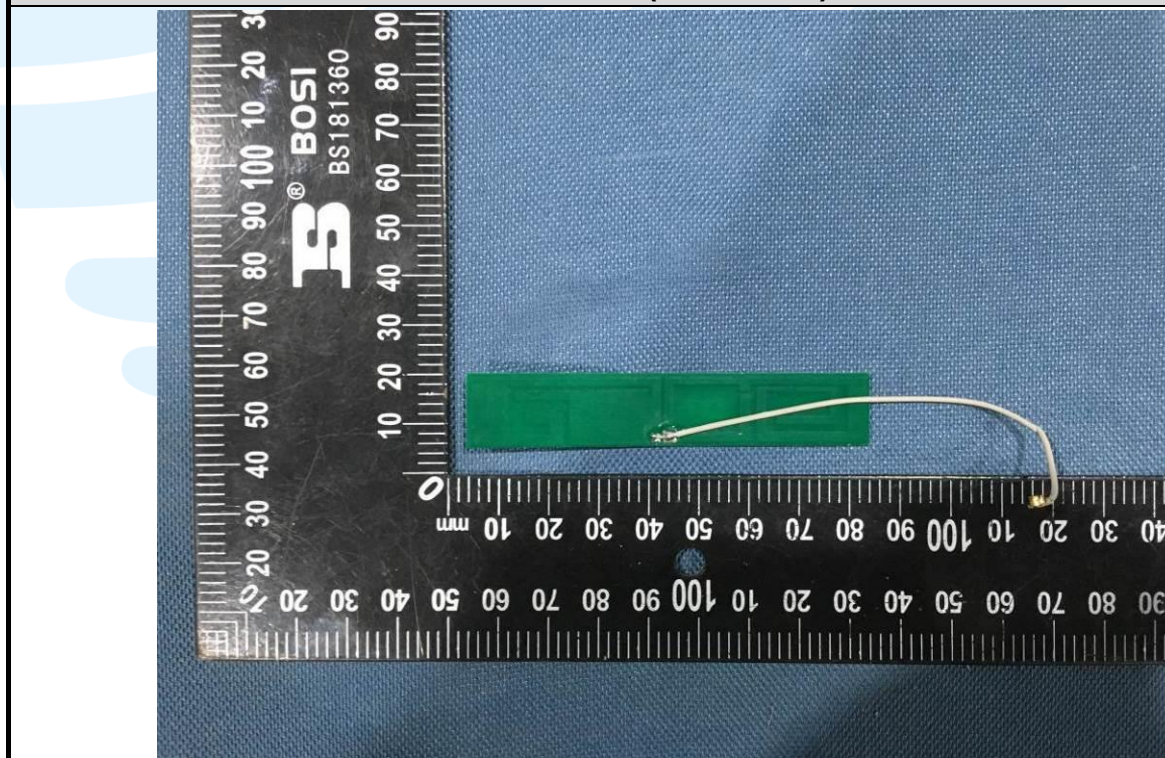
EUT Photo (Aux Antenna)
