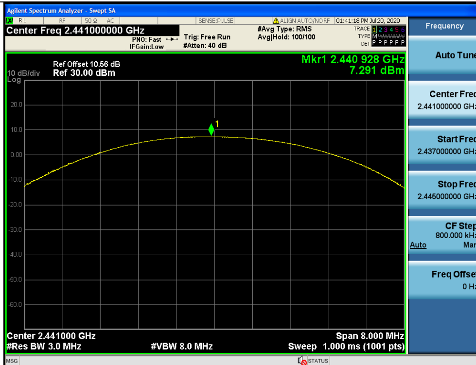
DH5_Ant1_2441
