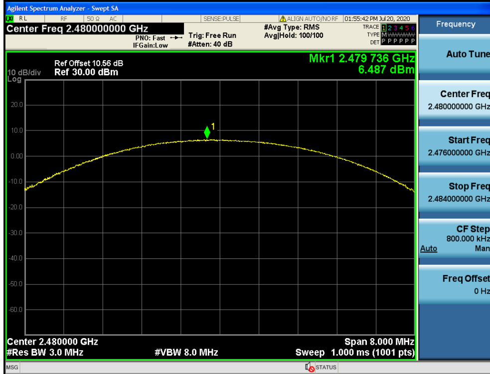
2DH5_Ant1_2480
