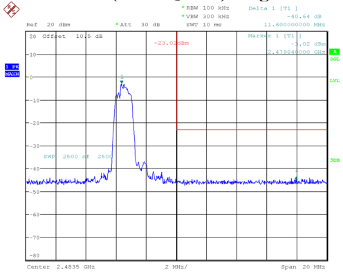
EDR ( \pi/4 -DQPSK): Right Side
