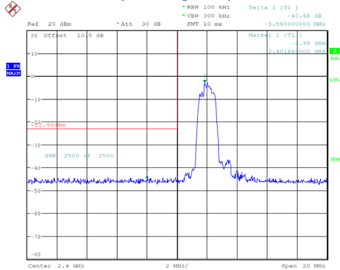
EDR ( \pi/4 -DQPSK): Left Side
