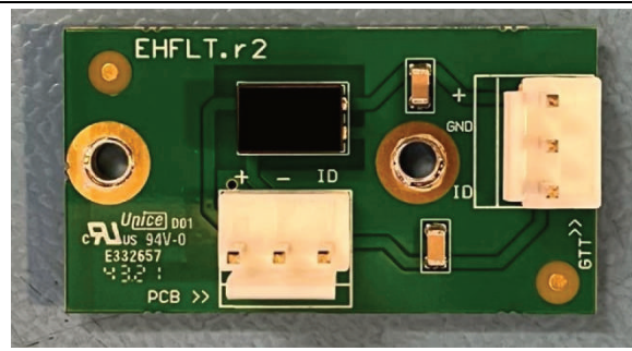
EHFLT (top)
