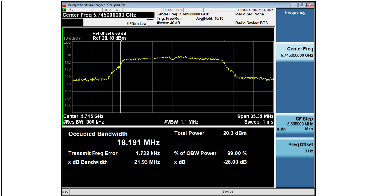
-26BW NVNT ANT1 802 11n(HT20) 5745
