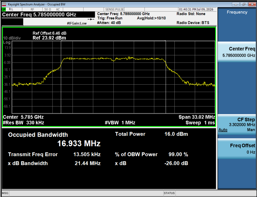
-26BW NVNT ANT1 802 11a 5785
