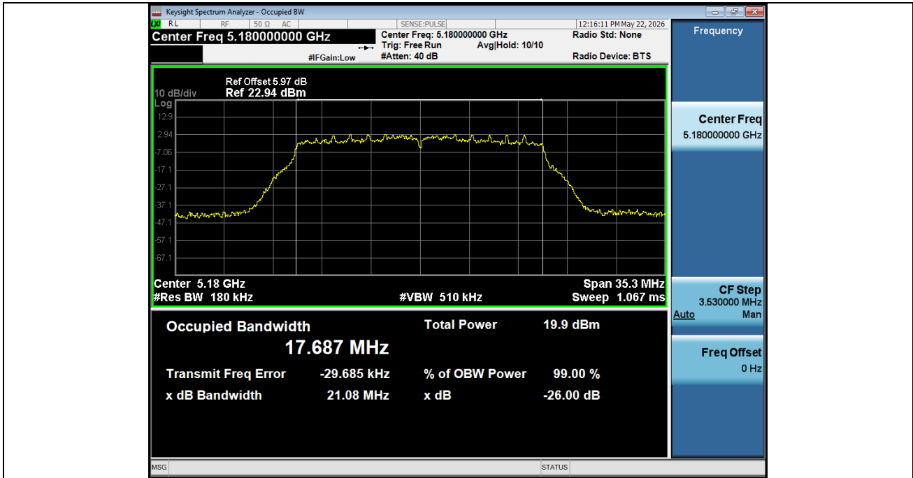
-26BW NVNT ANT2 802 11n(HT20) 5180
