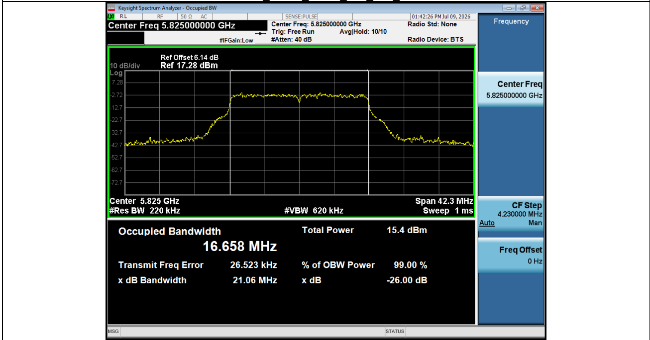
99%_OCB_NVNT_ANT2_802_11a_5825
