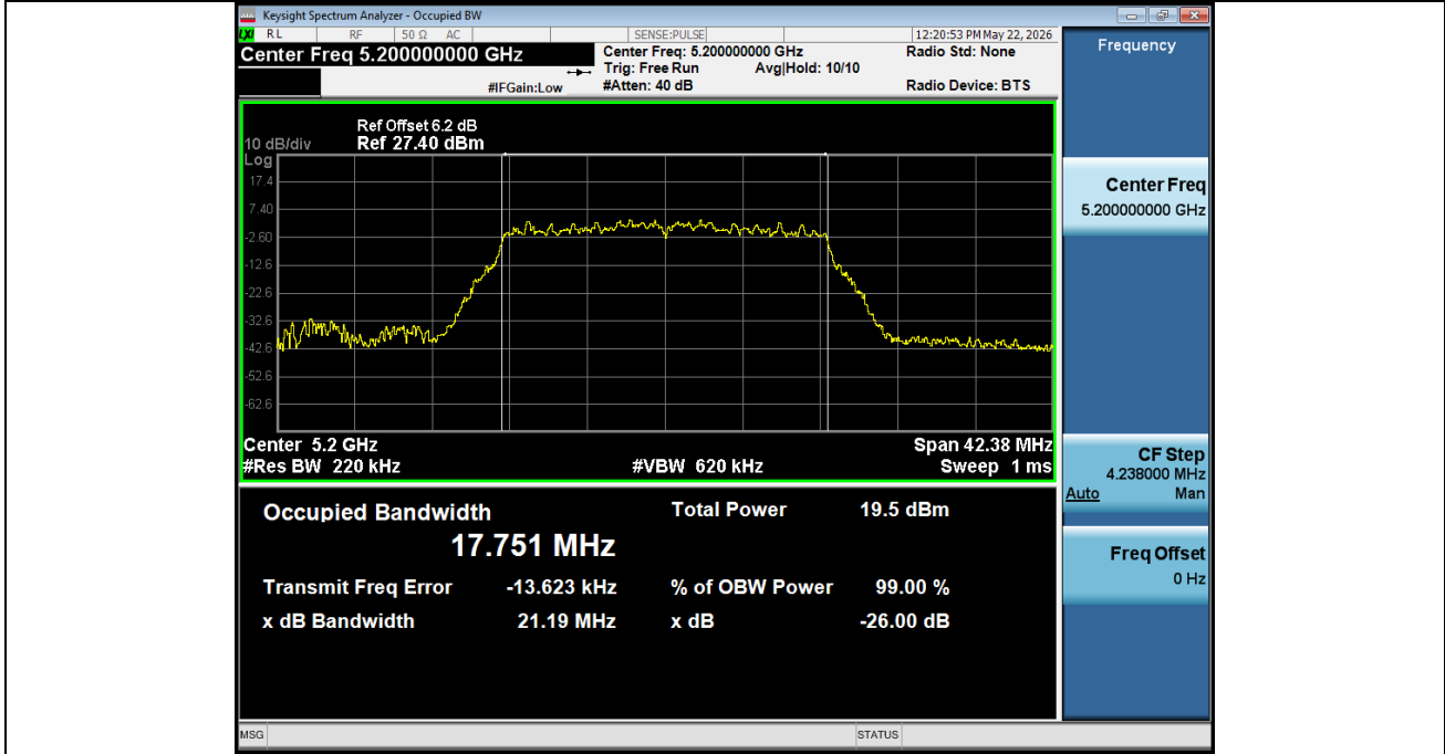
-26BW NVNT ANT2 802 11n(HT20) 5200
