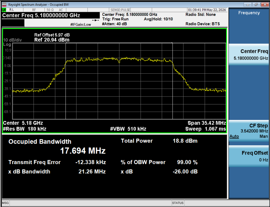
-26BW NVNT ANT1 802 11ax(HE20) 5180
