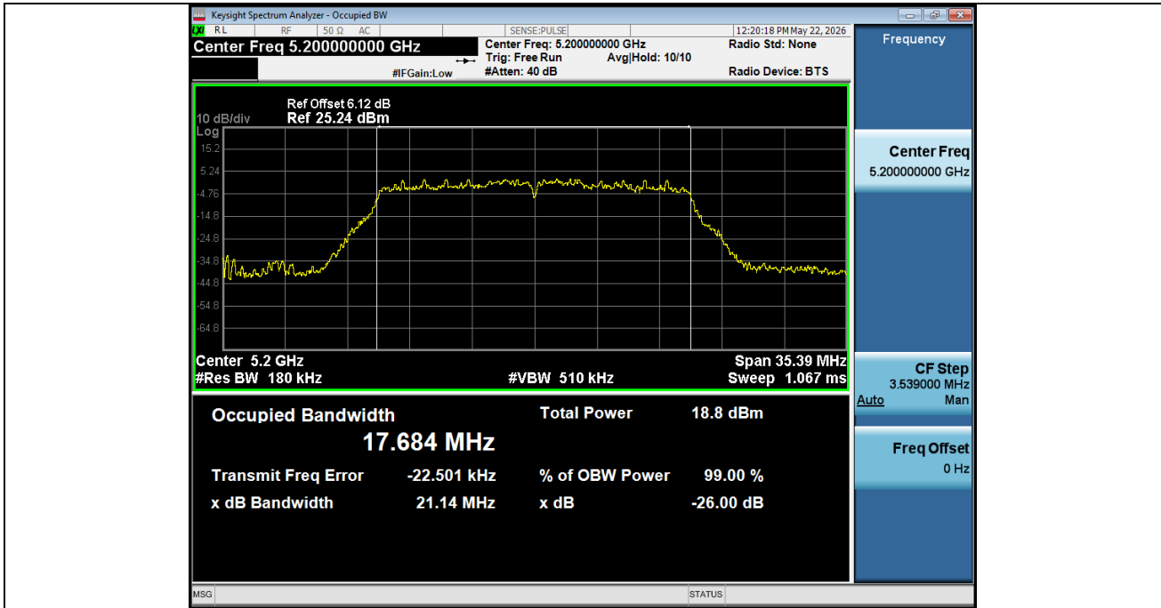
-26BW NVNT ANT1 802 11n(HT20) 5200
