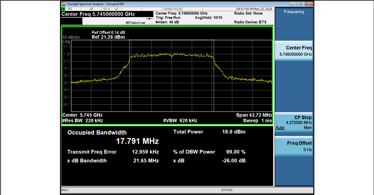
-26BW NVNT ANT2 802 11n(HT20) 5745
