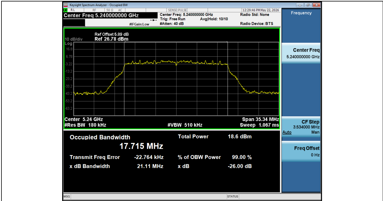
-26BW NVNT ANT2 802 11n(HT20) 5240
