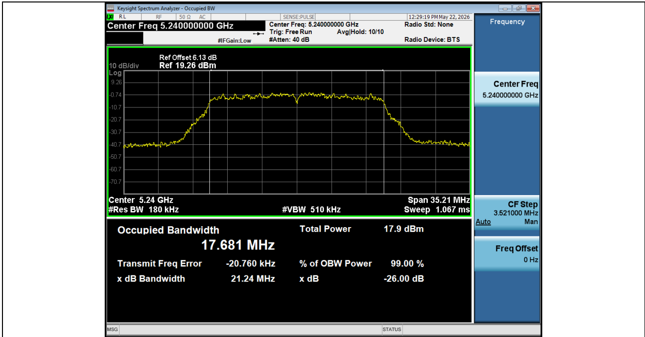
-26BW NVNT ANT1 802 11n(HT20) 5240
