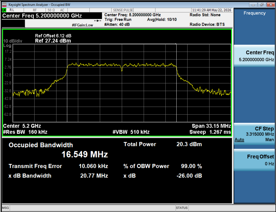
-26BW NVNT ANT1 802 11a 5200
