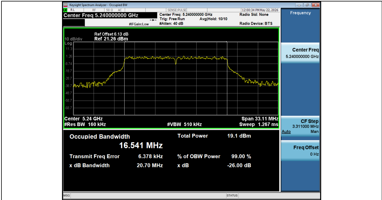
-26BW NVNT ANT1 802 11a 5240
