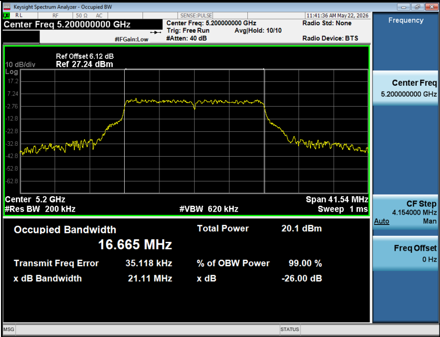
99%_OCB_NVNT_ANT2_802_11a_5200
