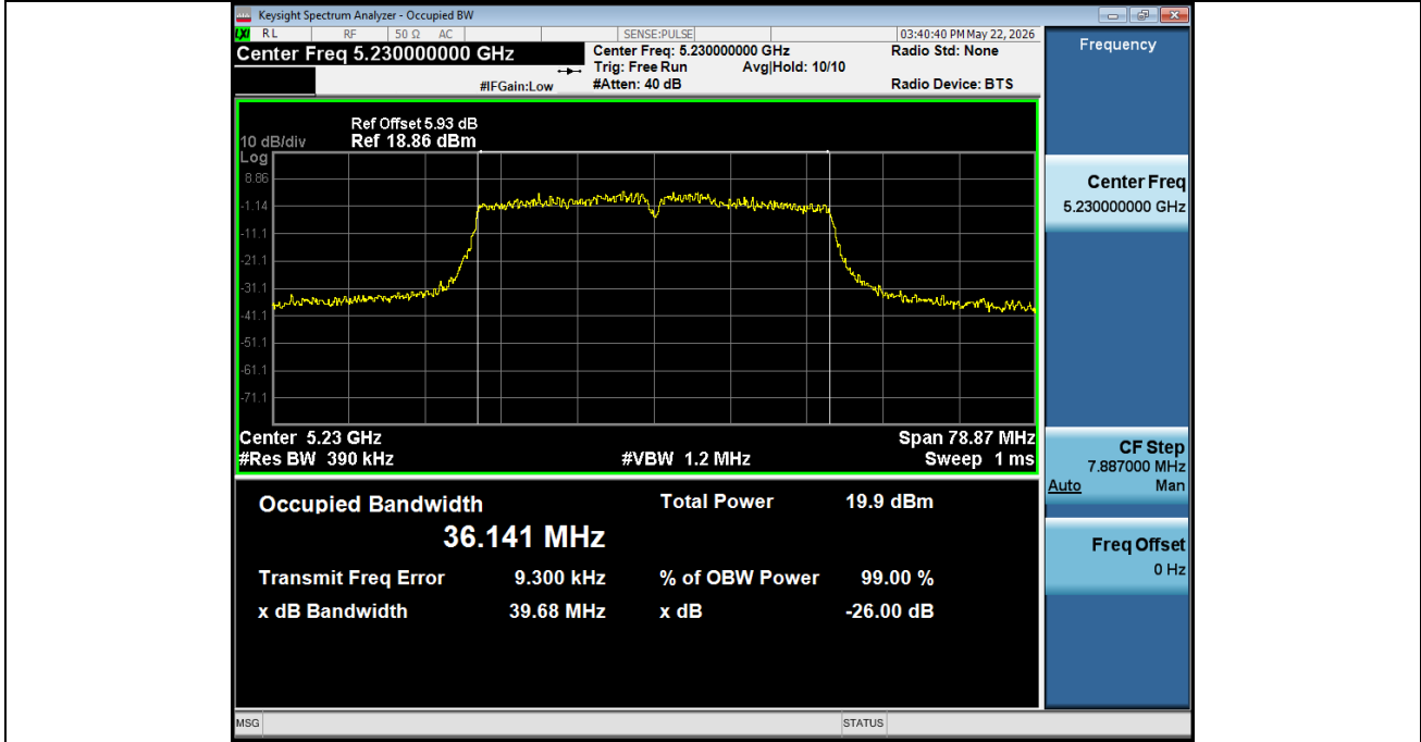
-26BW NVNT ANT2 802 11n(HT40) 5230
