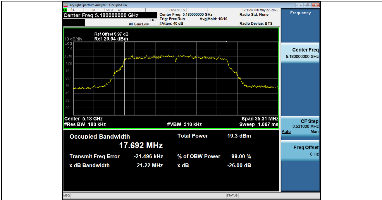
-26BW NVNT ANT1 802 11n(HT20) 5180
