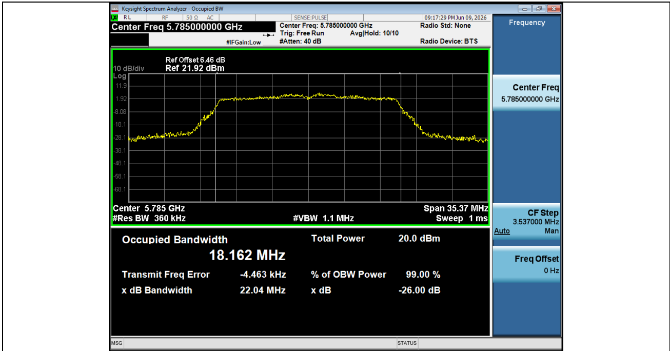
-26BW NVNT ANT1 802 11n(HT20) 5785
