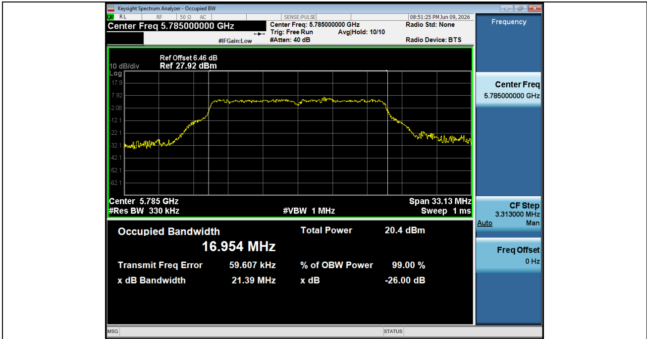
-26BW NVNT ANT1 802 11a 5785
