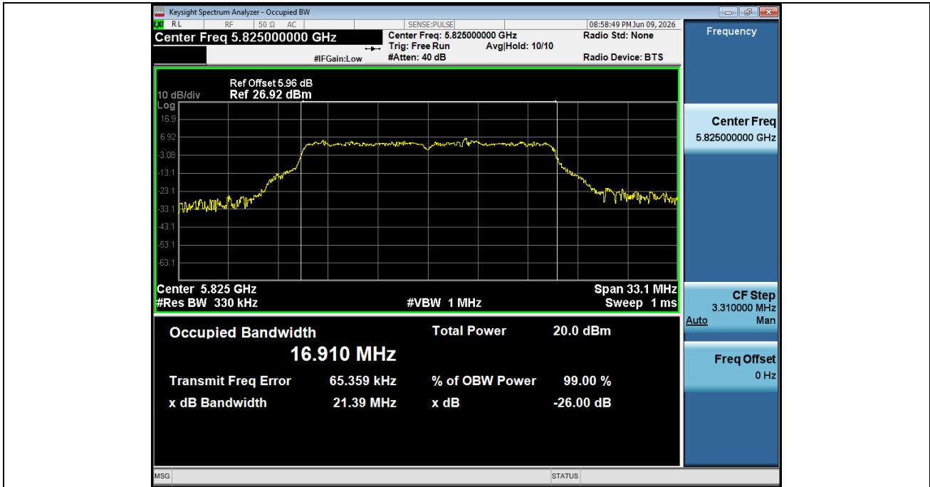
-26BW NVNT ANT2 802 11a 5825
