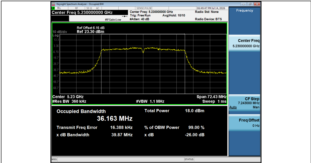
-26BW NVNT ANT1 802 11n(HT40) 5230
