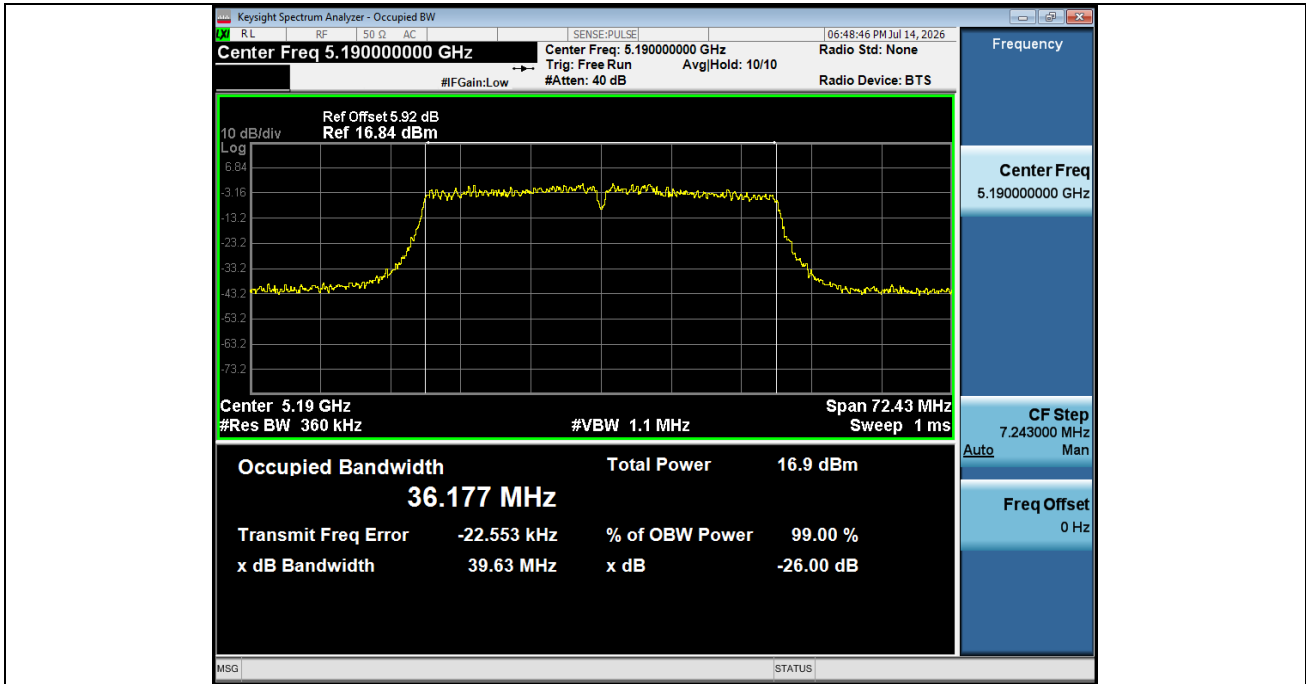
-26BW NVNT ANT2 802 11n(HT40) 5190
