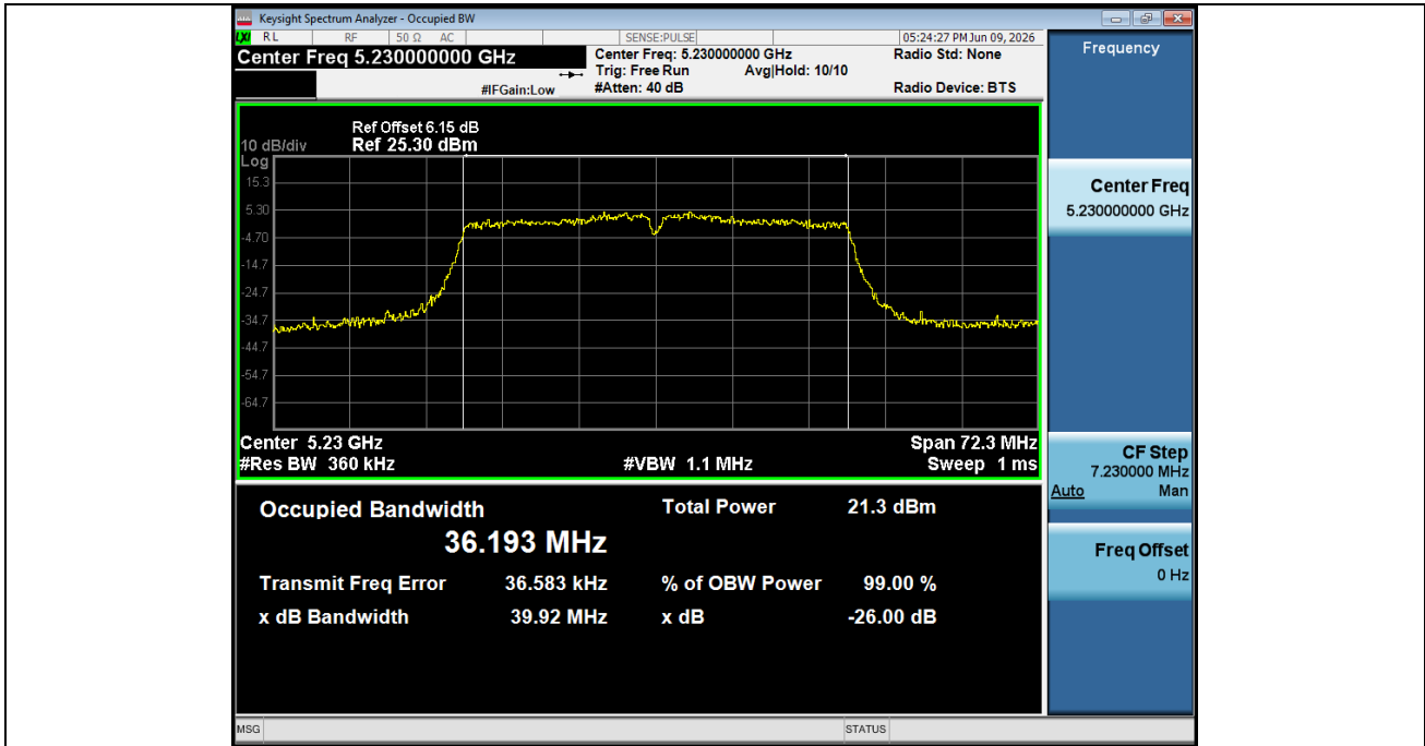
-26BW NVNT ANT1 802 11ax(HE40) 5230
