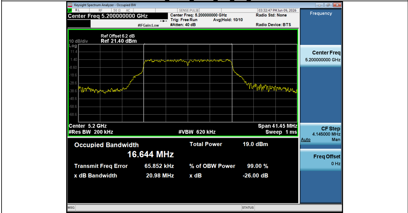
-26BW NVNT ANT2 802 11a 5200
