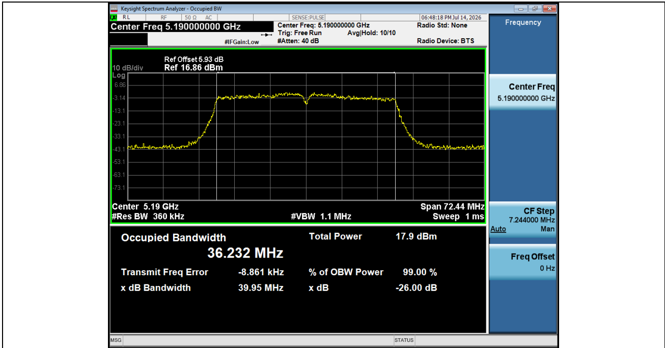
-26BW NVNT ANT1 802 11n(HT40) 5190
