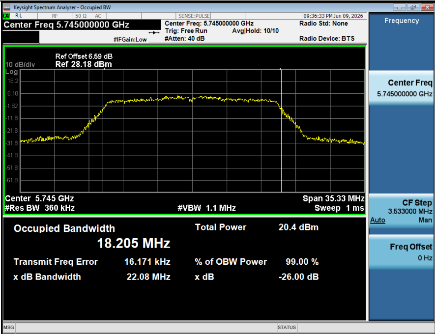
-26BW NVNT ANT1 802 11n(HT20) 5745
