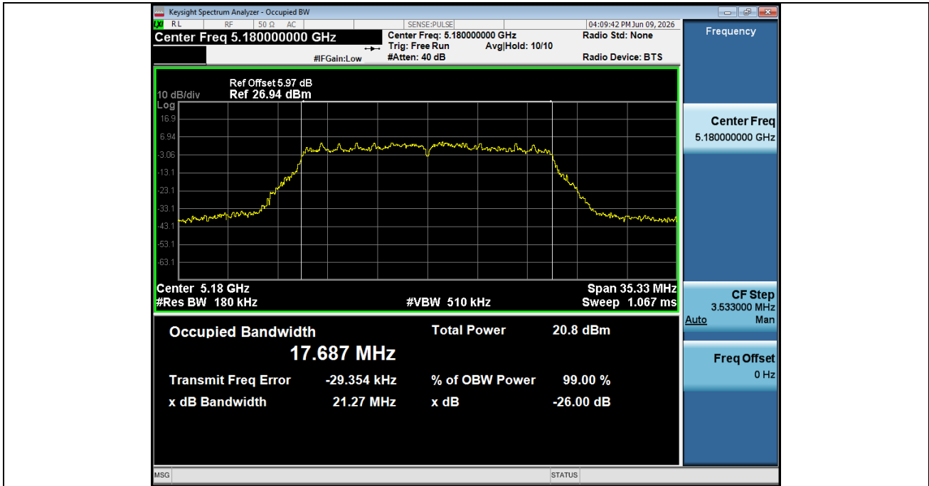
-26BW NVNT ANT1 802 11ax(HE20) 5180
