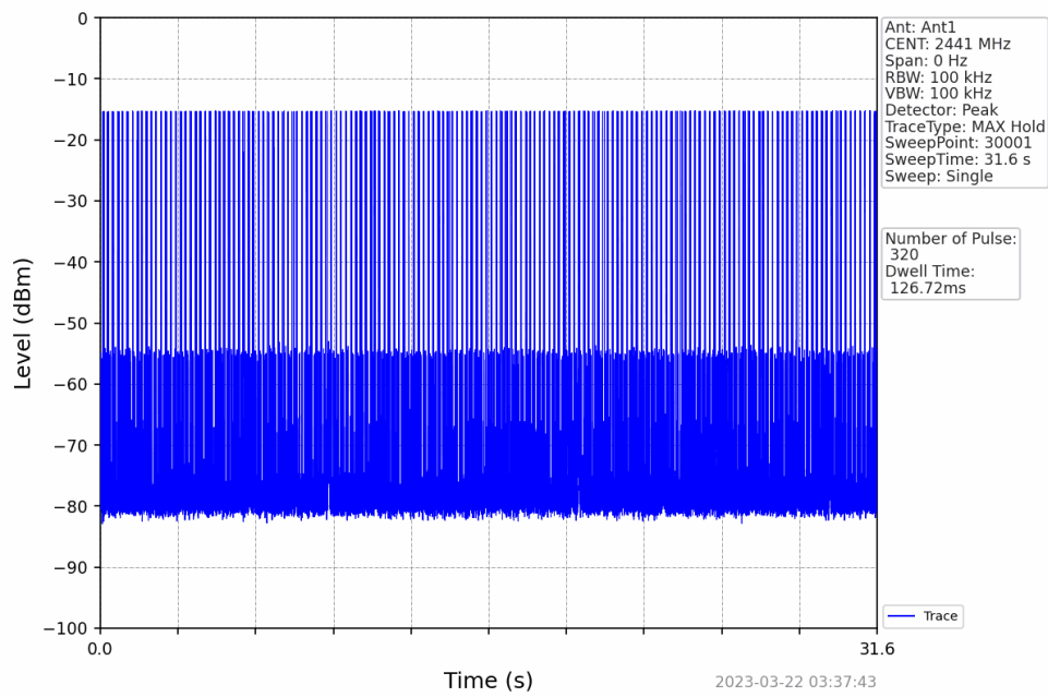
Pi/4DQPSK_2DH3_HOPP_Ant1_NTNV
