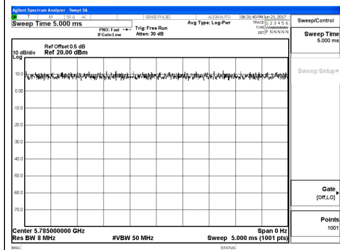
n20-5785MHz
