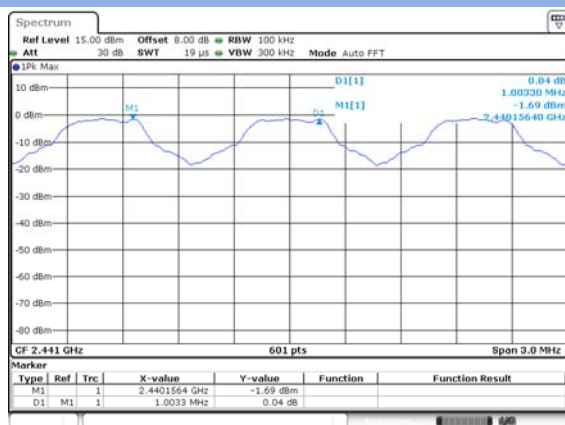
GFSK
