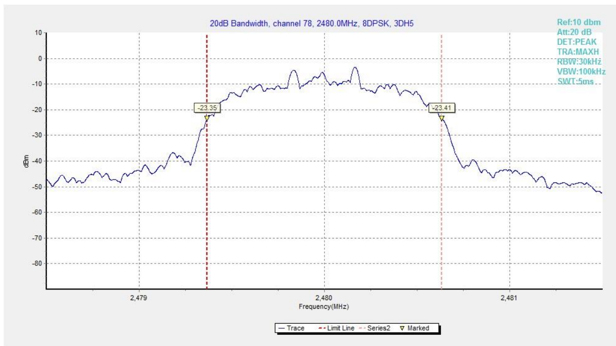
Fig. 107 20dB Bandwidth (8DPSK, Ch 78)
