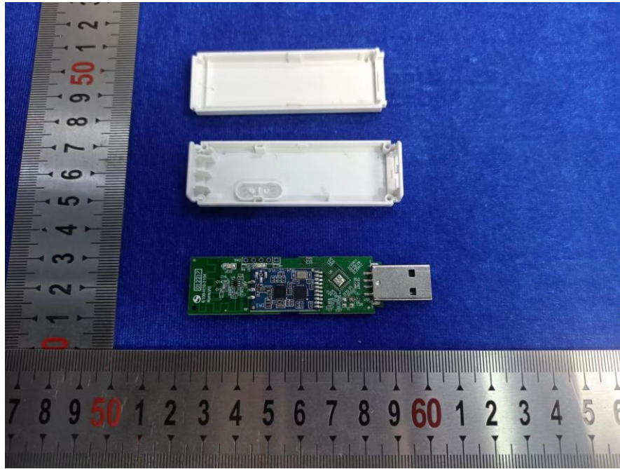
EUT-1
