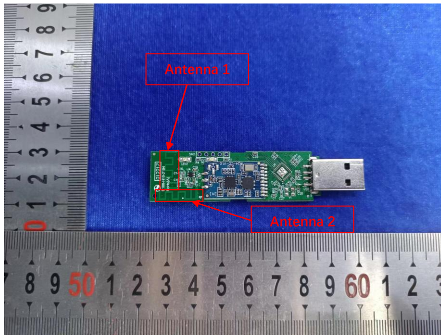
EUT-3
