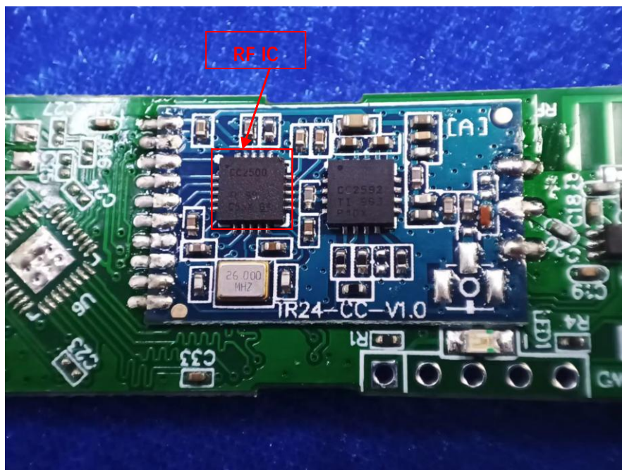
EUT-4
